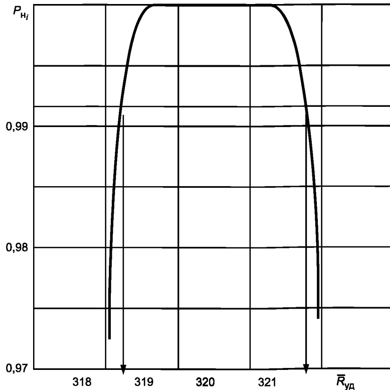
Рисунок В.1 — Зависимость P_{H_i} от \bar{R}_{y_{д}}
