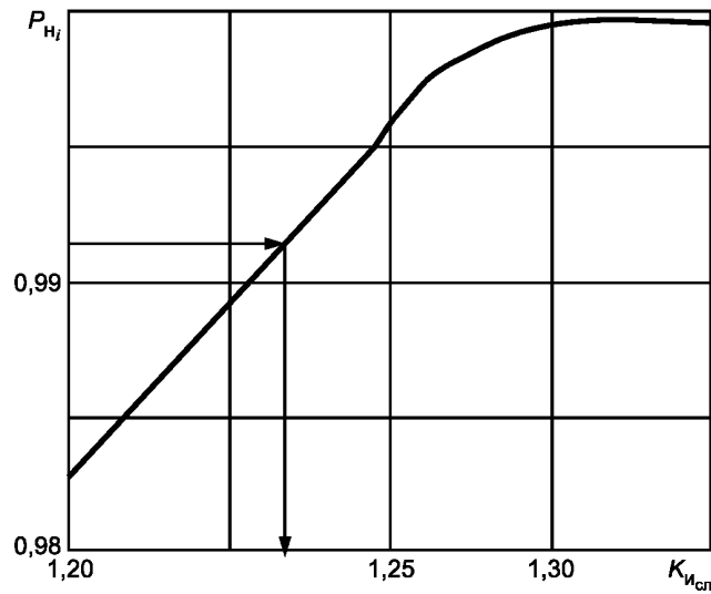
Рисунок В.2 — Зависимость P_{H_i} от K_{исл}
