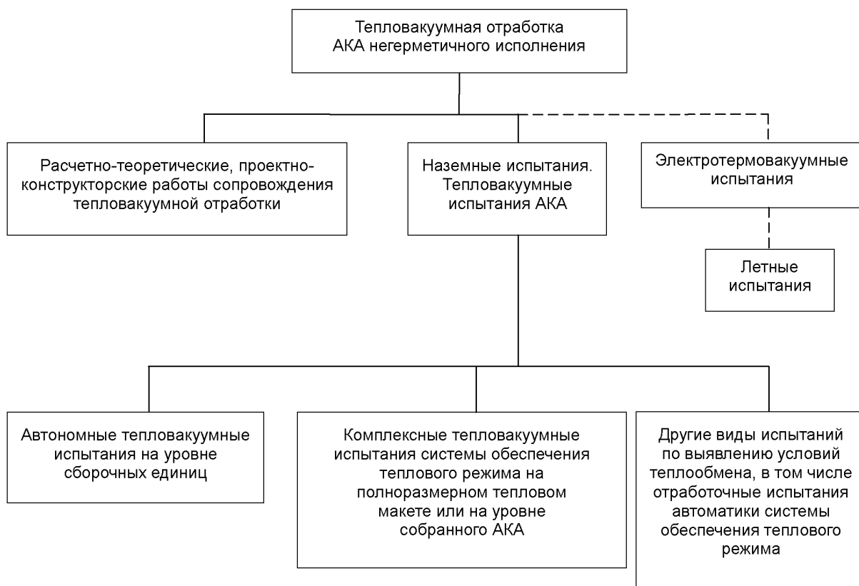
Рисунок А.1
