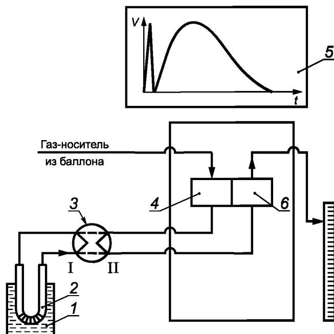
1 — стакан вместимостью 250 см 3 по ГОСТ 25336; 2 — U-образная стеклянная трубка с внешним диаметром 5 мм, высотой 100 мм, расстоянием между концами 35 мм; 3 — четырехходовой кран; 4 — сравнительная ячейка детектора; 5 — самописец; 6 — измерительная ячейка детектора
