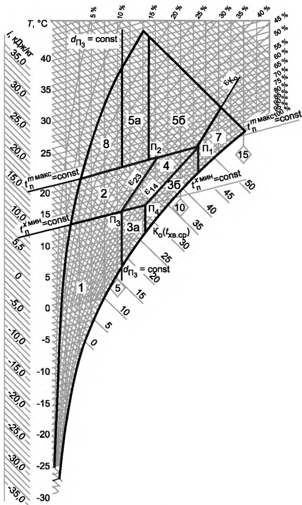
Рисунок 3 — Деление на погодные зоны области возможных сочетаний энтальпии и влагосодержания наружного воздуха для ЦСКВ с парувлажителем
