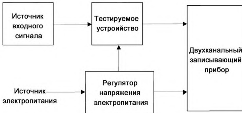
Рисунок 1 – Схема проведения испытаний для определения влияния понижения напряжения электропитания или его кратковременного отключения
