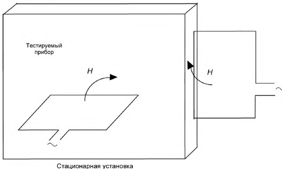
Рисунок 3b – Пример применения тестового магнитного поля с помощью метода приближения
