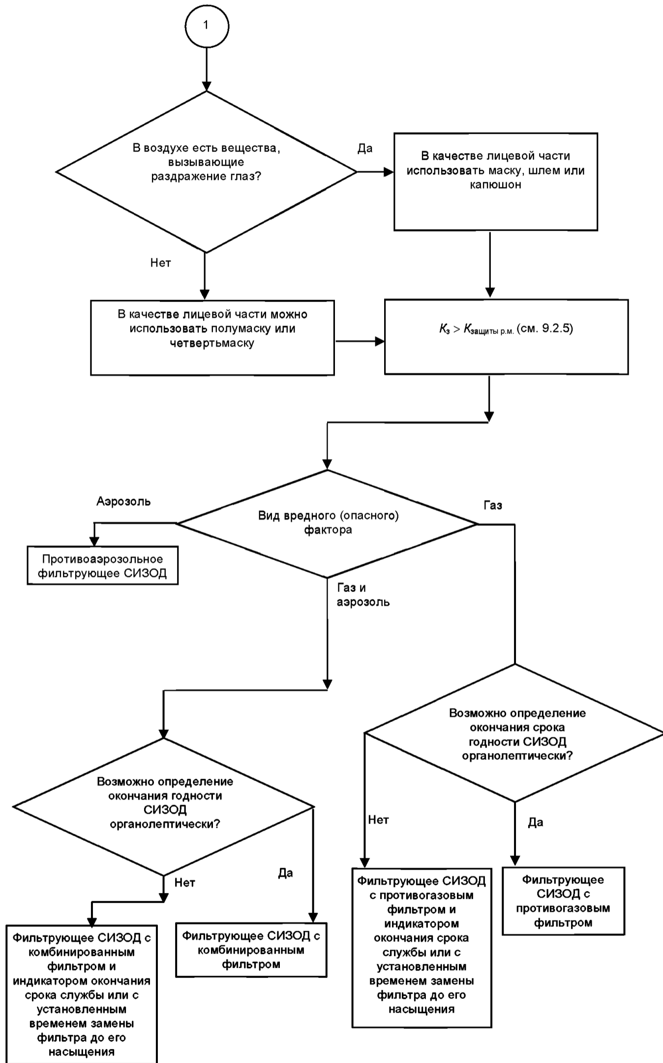
Рисунок В.1 — Алгоритм выбора СИЗОД
