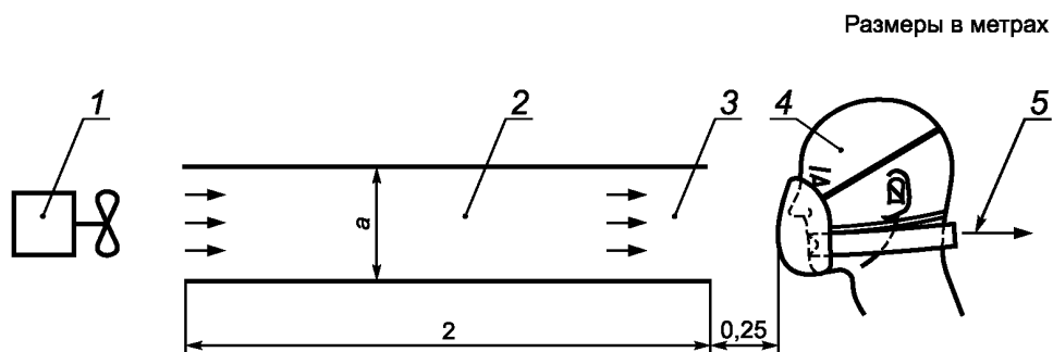
1 — вентилятор; 2 — трубопровод; 3 — датчик воздушного потока; 4 — голова манекена; 5 — по направлению к дыхательной машине; размер a — 0,3 — 0,5 м
