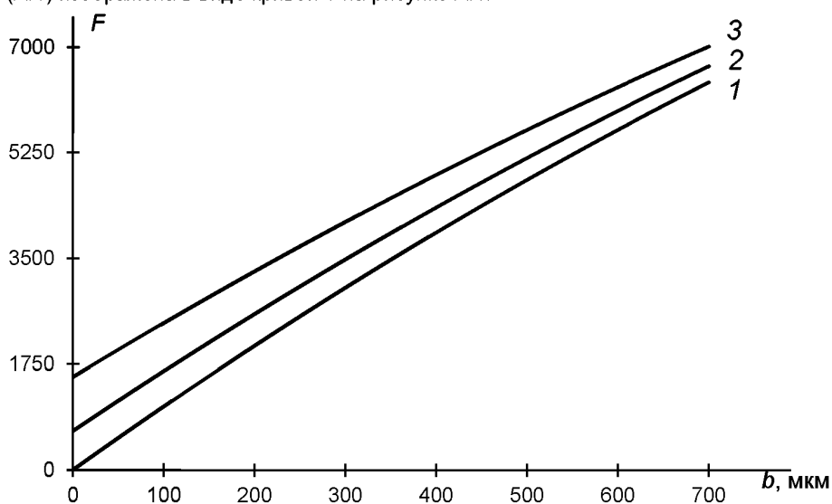
Рисунок А.1 — Зависимость сигнала F от толщины b при разной толщине s (преобразователь с оптимизированными характеристиками)
