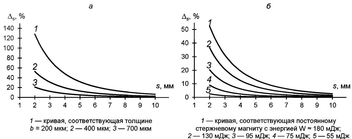
Рисунок 3 — Зависимость дополнительной погрешности \Delta_s , обусловленной намагниченностью корпуса камеры, от толщины s :
