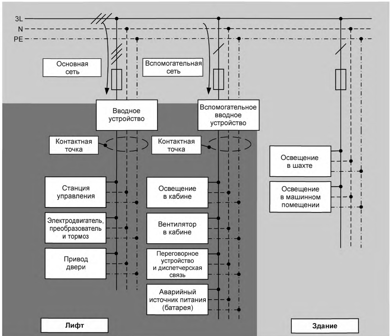
Рисунок А.1 — Подключение средств измерения энергопотребления лифтов
