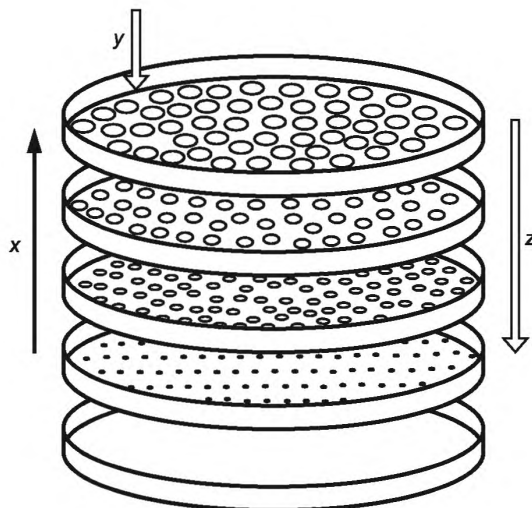
Рисунок 1 — Схема устройства для ситового анализа
