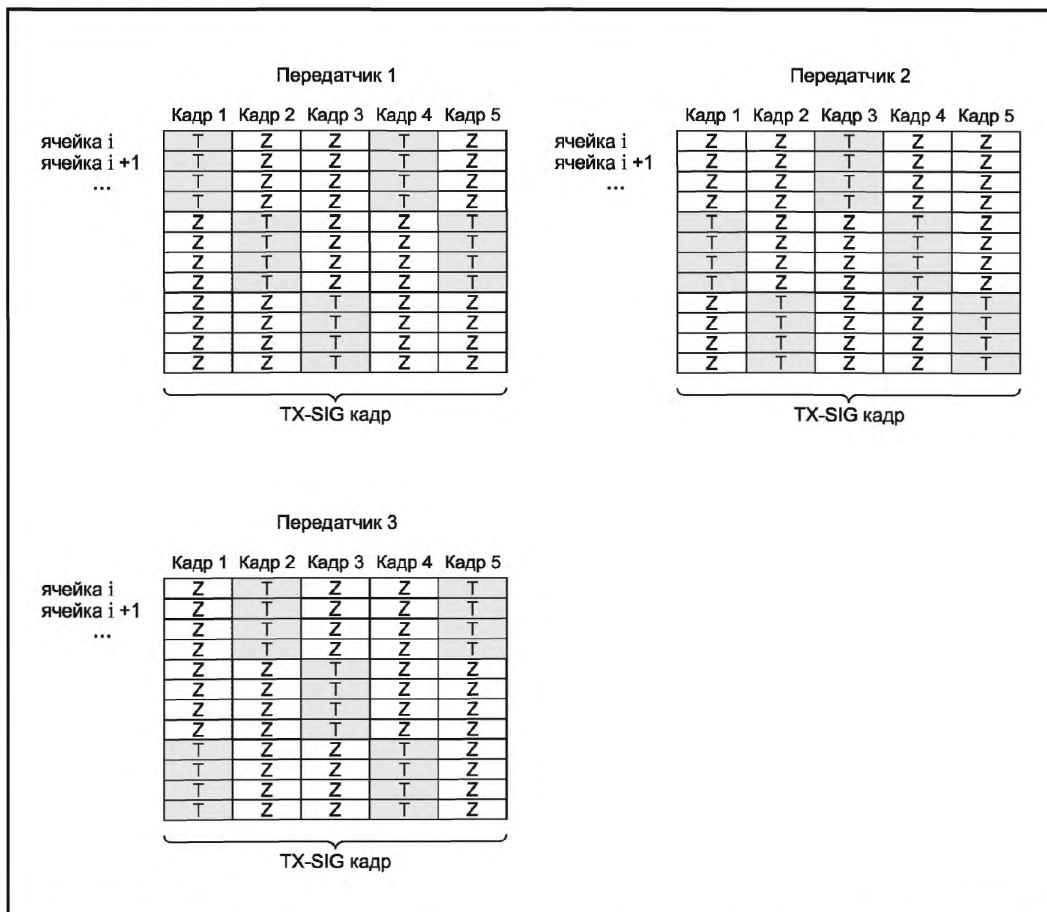
Рисунок 1 — Пример шаблонов дополнительных ячеек, содержащих сигнатуры передатчиков, перед вставкой B-ячеек, для случая M = 3, N = 4, L = 5
