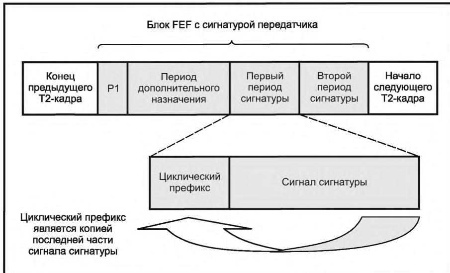
Рисунок 3 — Структура блока FEF с сигнатурой передатчика
