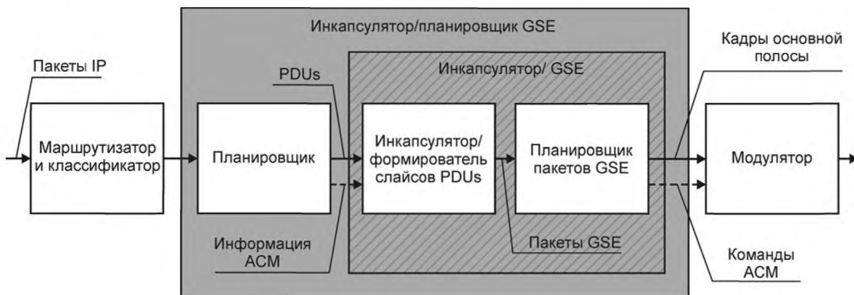
Рисунок А.1 — Блок-схема инкапсулятора и планировщика
