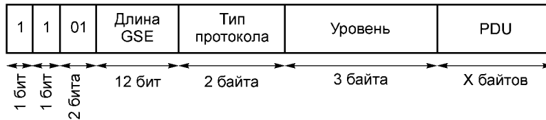
Рисунок В.2 — Пакет GSE, переносящий полный нефрагментированный PDU с 3-байтовым адресом NPA
