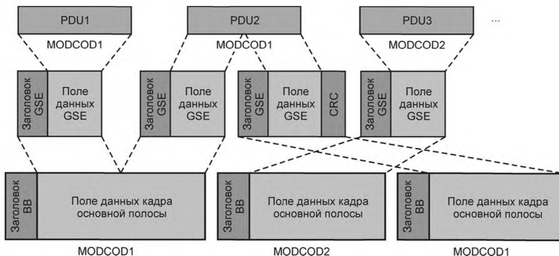
Рисунок А.3 — Совмещенные операции инкапсуляции и планирования
