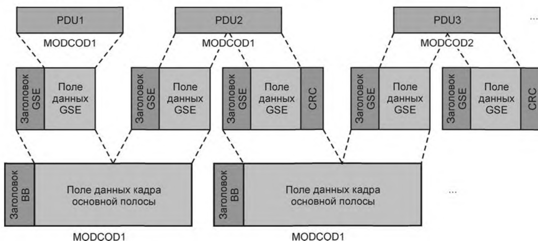
Рисунок А.2 — Несомещенные операции инкапсуляции и планирования
