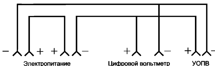
Рисунок 2 — Схема подключения цифрового вольтметра
