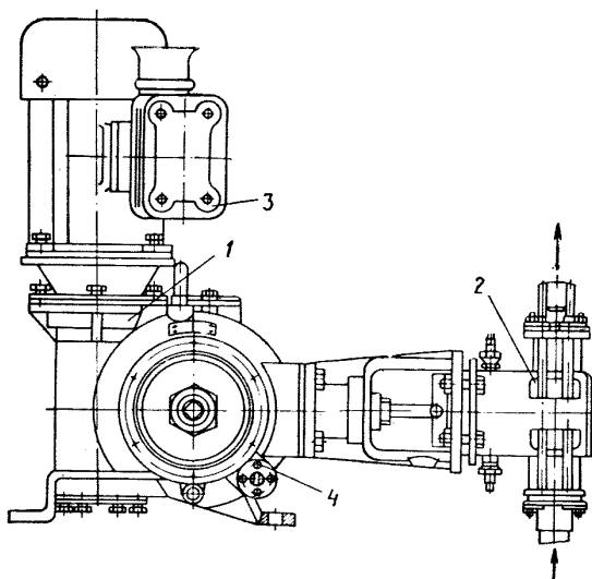
Рис. 4. Насос-дозатор серии НД для смолизации прунтов 1 — редуктор; 2 — гидравлическая часть; 3 — электродвигатель; 4 — регулятор подачи жидкости
