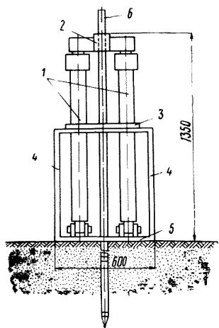
Рис. 2. Устройство для извлечения инъекторов
