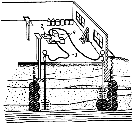
Рис. 7. Схема опытного определения интенсивности поглощения раствора грунтом
