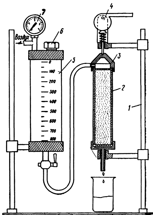
Рис. 8. Прибор для лабораторного закрепления грунтов
