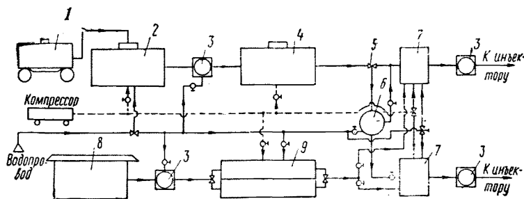
Рис. 5. Технологическая схема приготовления и заправки реагентов 1 — цистерна с концентрированной кислотой; 2 и 4 — емкости для приготовления и расхода рабочего раствора кислоты; 3 — насосы; 5 — трехходовой кран; 6 — дозатор рабочего раствора кислоты; 7 — дозаторы гелеобразующего раствора; 8 — склад со смолой; 9 — двоякая емкость для приготовления и расхода рабочего раствора смолы
