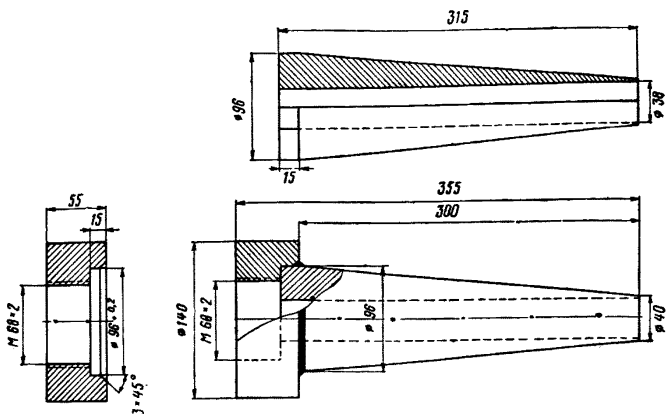
Рис. 6. Устройство для тампонажа устья инъекционной скважины
