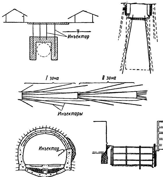
Рис. 1. Расположение инъекторов при закреплении выработок
