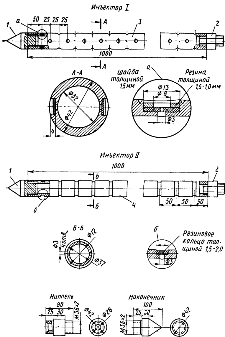
Рис. 3. Инъекторы I и II для смолизации песчаных грунтов 1 — наконечник; 2 — ниппель; 3 и 4 — перфорированные звенья
