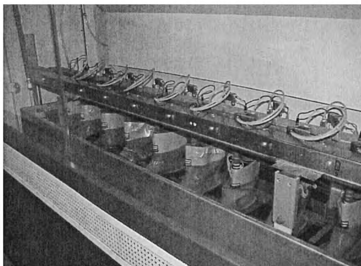
Рисунок 2 — Типовая аппаратура для определения диэлектрических свойств резиновой обуви с использованием воды в качестве электродов
