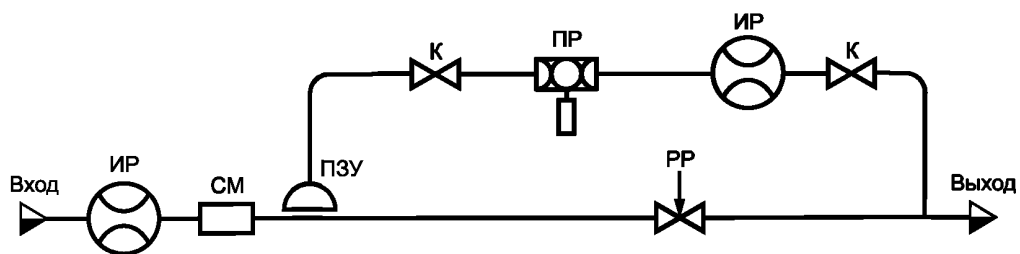
Рисунок А.4 — Средства отбора проб сырой нефти из потока нефтегазовой смеси, расположенные в трубопроводе
