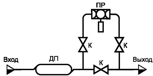
Рисунок А.6 — Средства отбора проб сырой нефти из потока нефтегазовой смеси, расположенные в трубопроводе с депульсатором на входе
