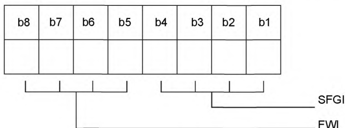
Рисунок 7 – Кодирование байта интерфейса ТВ(1)
