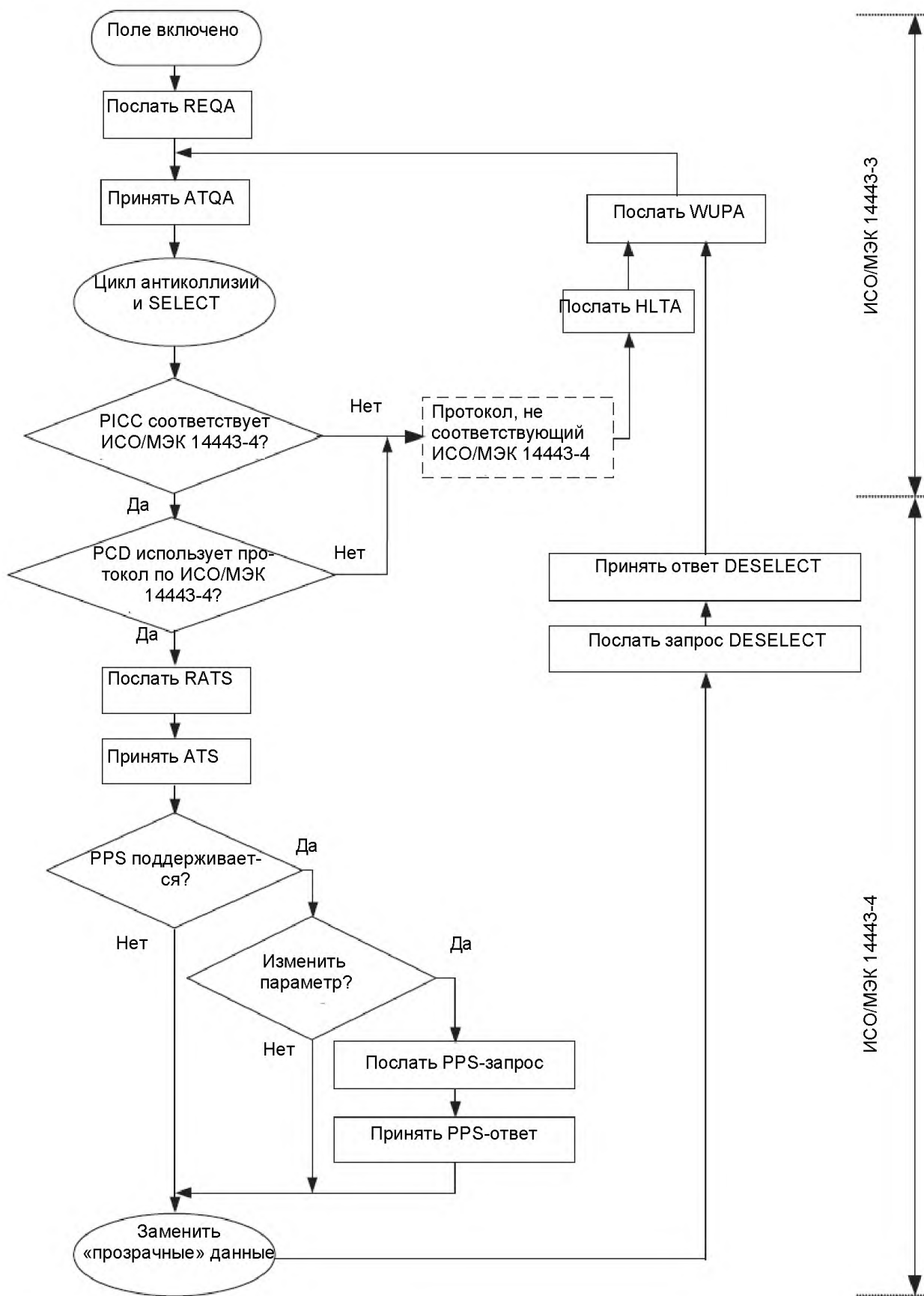
Рисунок 1 – Активация PICC типа А с помощью PCD
