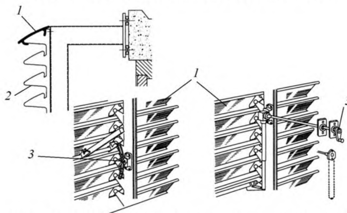
Рисунок 7 – Горизонтальные регулируемые жалюзи
