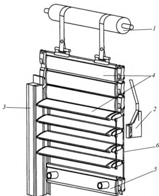
Рисунок 6 – Горизонтальные регулируемые жалюзи
