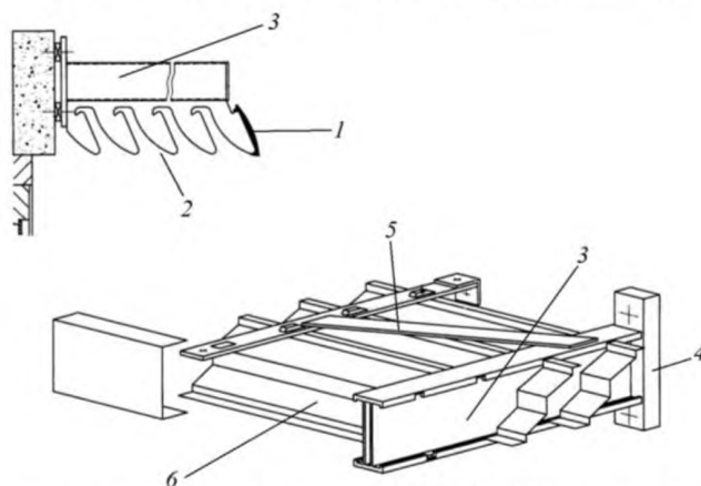
Рисунок 7 – Горизонтальные регулируемые жалюзи
