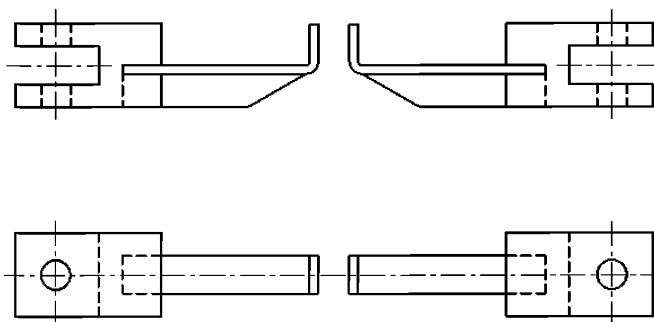
Рисунок 1 – Держатели образца для испытаний
