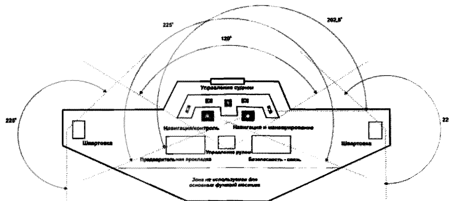
Рис. 2.5.17-1 Расположение рабочих постов и требуемые зоны видимости для них. Определение местоположения на бумажных картах — проход и место управления судном впереди
