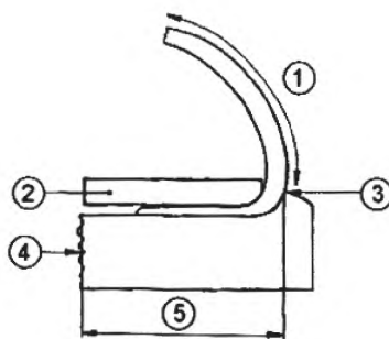
1 – ~ 15; 2 – стелька (удаленная); 3 – линия затыжной кромки; 4 – подошва; 5 – ~ 15
