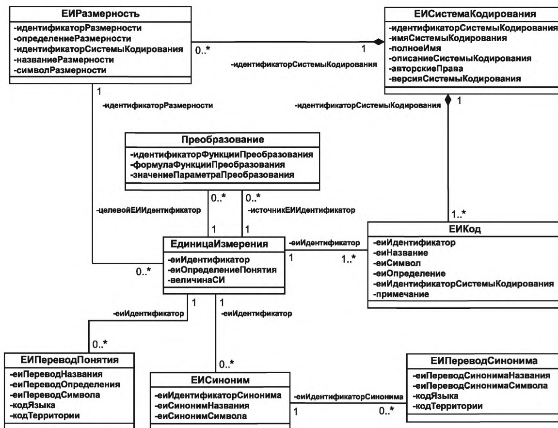
Рисунок 2 — Диаграмма классов UML для понятий единиц измерения
