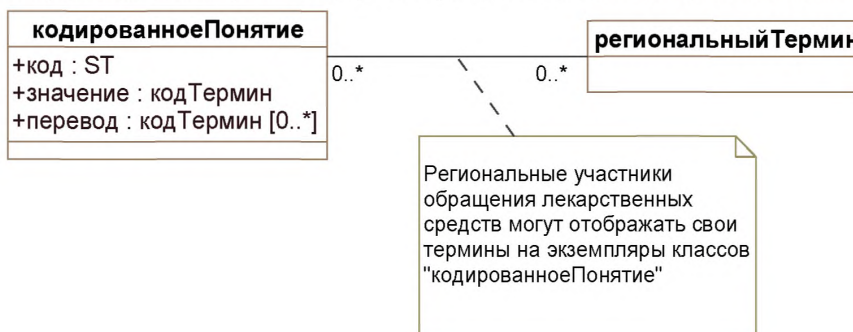
Рисунок 4 – Концептуальная диаграмма, указывающая цель процесса отображения
