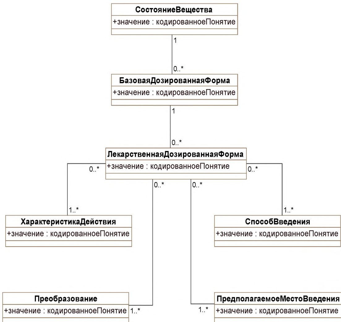
Рисунок 5 – Концептуальная диаграмма класса «ЛекарственнаяДозированнаяФорма»
