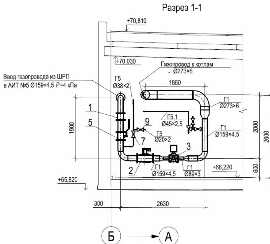
Рисунок В.2 – Пример выполнения разреза для котельной
