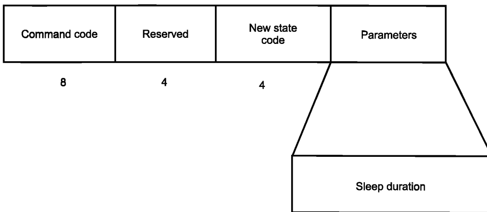
Рисунок 35 – Формат команды «Переключение в состояние «Энергосбережение» (SwitchState(Sleep))
