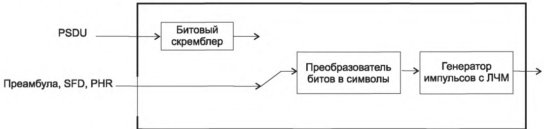
Рисунок 4 – Эталонный модулятор для двухточечной ортогональной ЛЧМ
