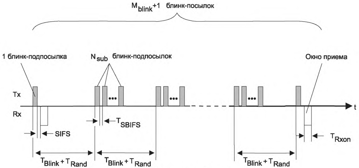
Рисунок 29 – Режим передачи блинк-посылки
