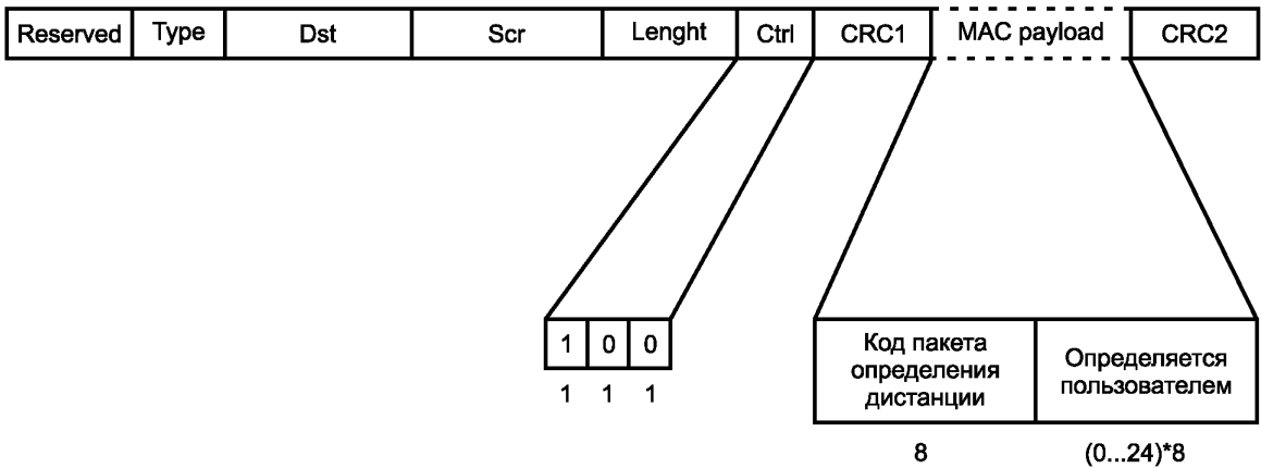
Рисунок 46 – Формат пакета измерения расстояния T1R1
