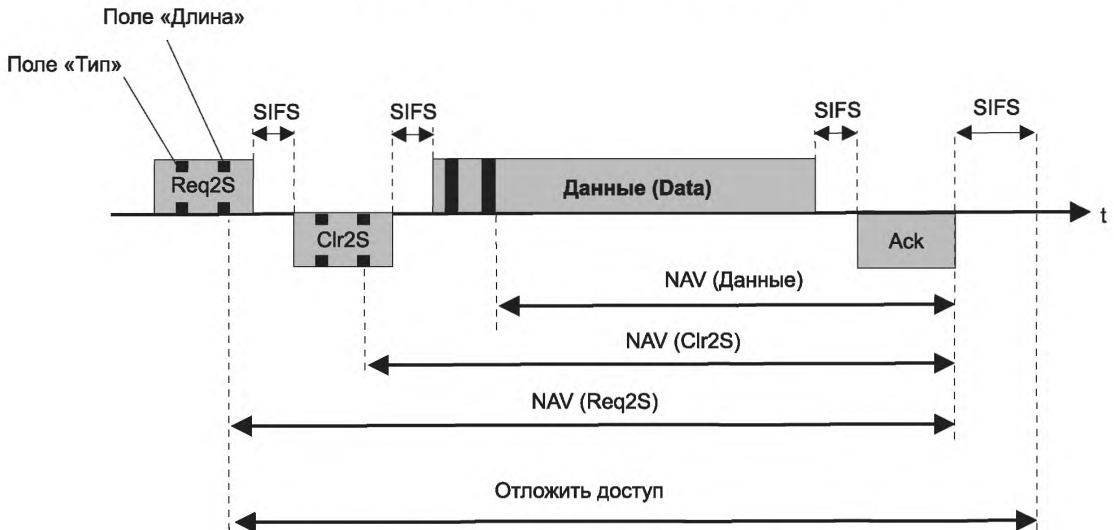
Рисунок 26 – NAV для трехэтапного установления связи
