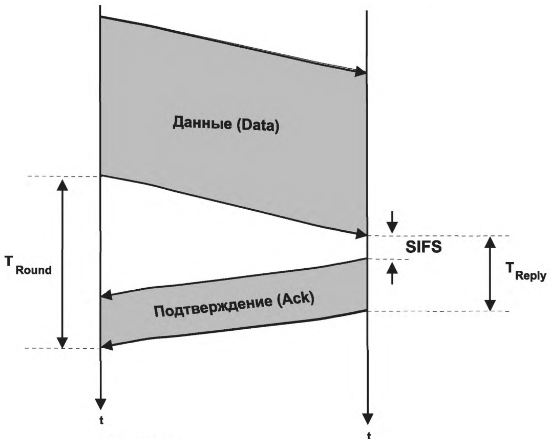
Рисунок 22 – Временные параметры подтверждения данных
