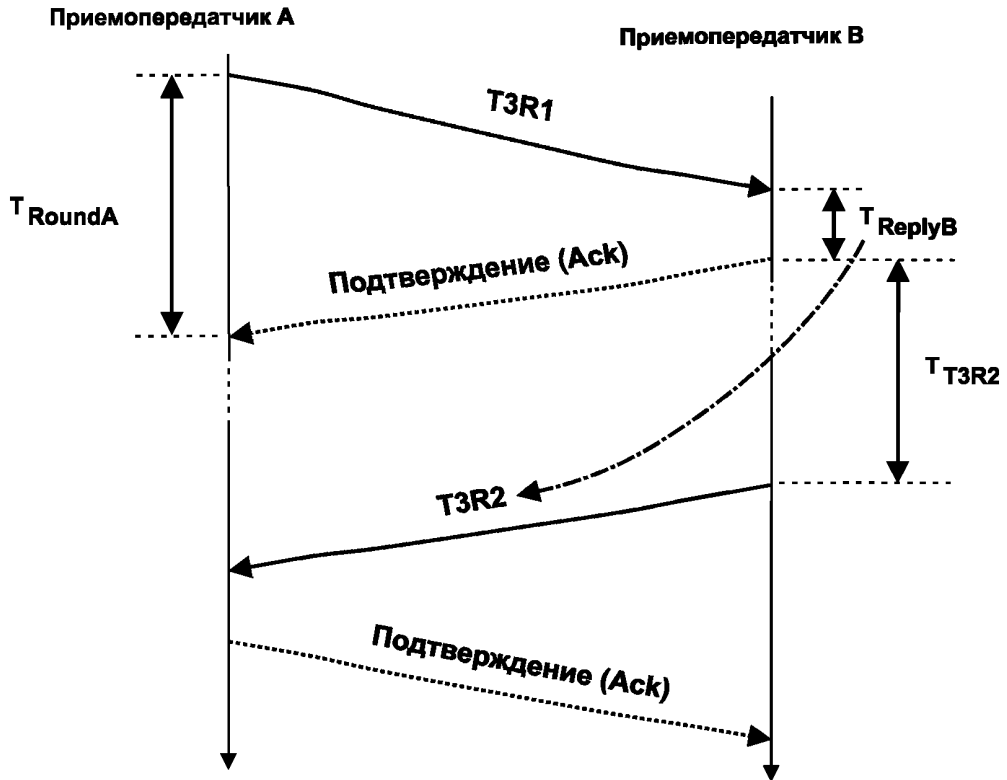
Рисунок 58 – Обмен пакетами измерения расстояния типа 3
