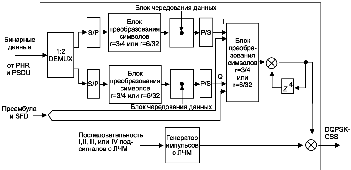
Рисунок 12 – Эталонный модулятор для DQPSK-CSS
