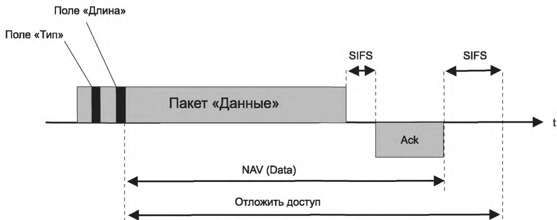
Рисунок 24 – NAV для пакетов «Данные» (Data)
