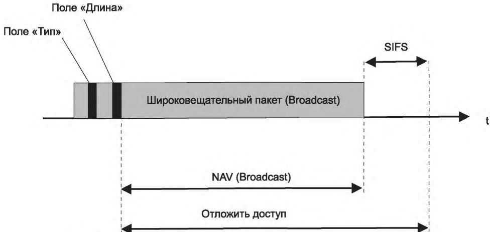
Рисунок 25 – NAV для пакетов «Широковещательный пакет» (Broadcast)
