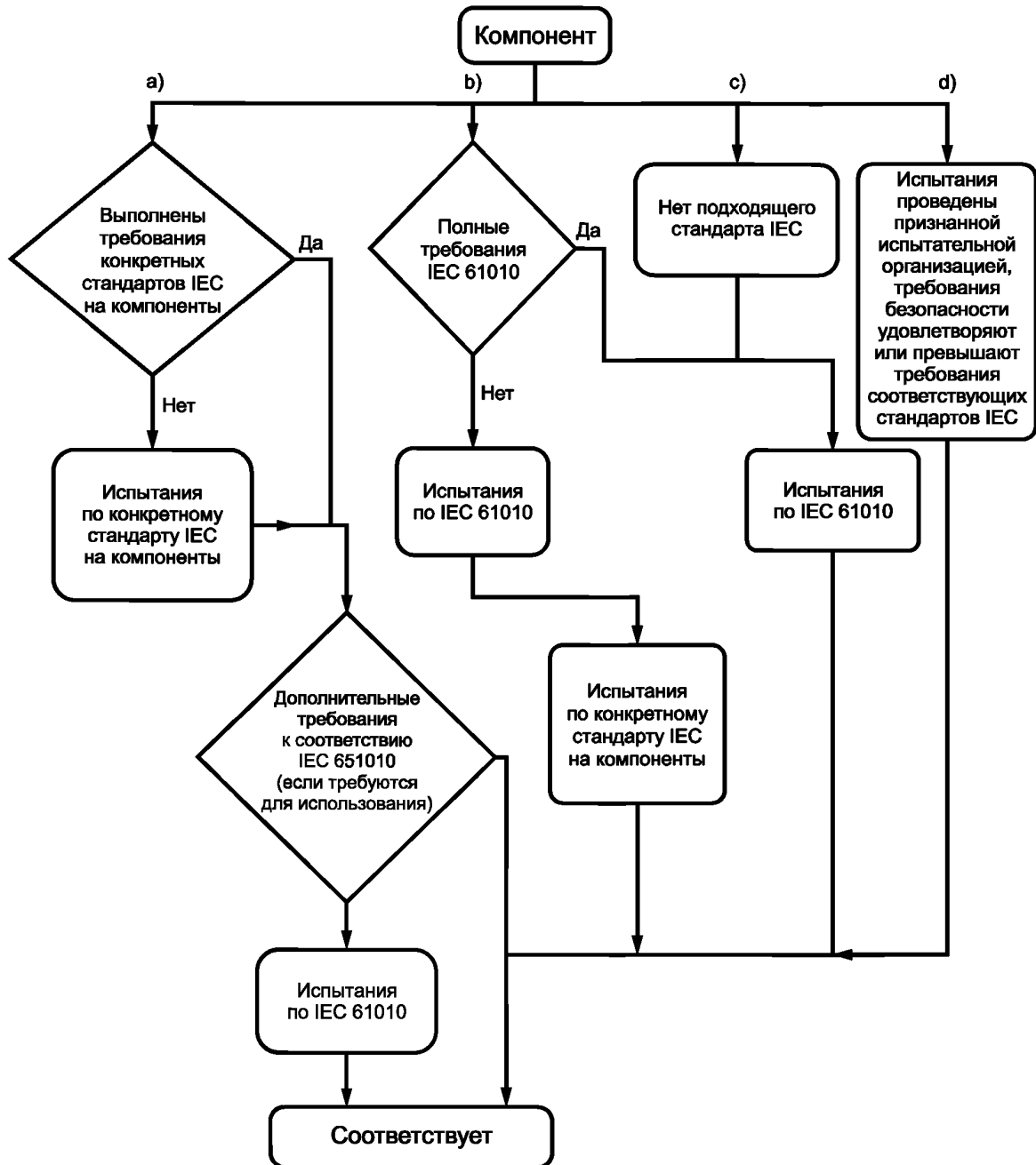
Рисунок 15 — Алгоритм вариантов проверки соответствия по 14.1, перечисления a), b), c) и d)
