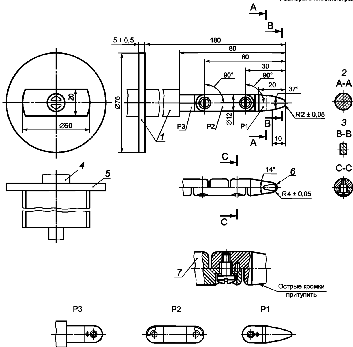
1 — изоляционный материал; 2 — разрез А-А; 3 — разрез В-В; 4 — рукоятка; 5 — стопорная пластина; 6 — сферический край; 7 — деталь х (пример)
