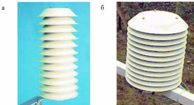
Рисунок 8.2 – Радиационная защита DTR 502 (а) и DTR 13 (б)
