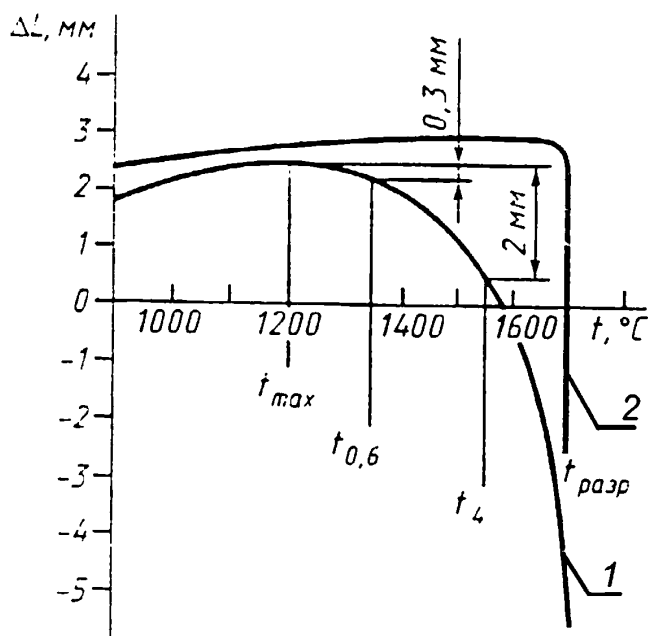
1 – для алюмосиликатных огнеупоров; 2 – для периклазовых огнеупоров.
