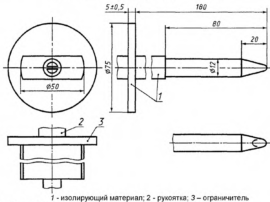
Рисунок Г.1 — Шарнирный испытательный палец
