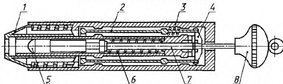
1 - выходной конус; 2 - стержень спускового механизма; 3 - пружина спускового механизма; 4 - спусковой кулачок; 5 - головка молотка; 6 - пружина молотка; 7 - шток; 8 - ручка для взвода пружины Рисунок Г.5 — Испытательный молоток
