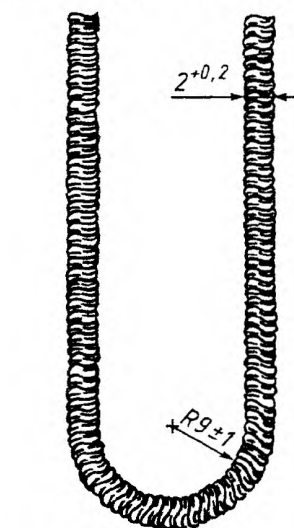
Рисунок Г.4 — Испытательная цепочка
