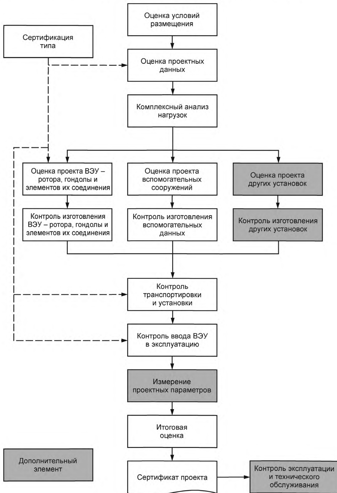
Рисунок 2 — Блок-схема процедуры сертификации проекта
