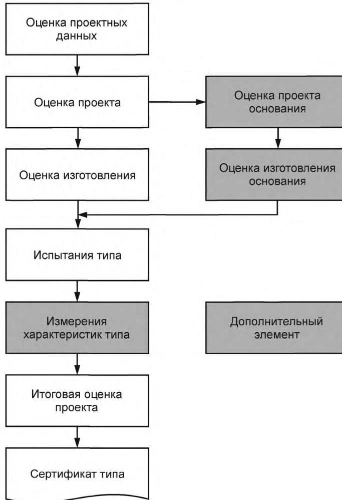
Рисунок 1 — Блок-схема процедуры сертификации типа
