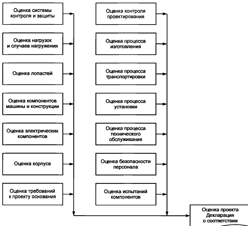
Рисунок 4 — Блок-схема процедуры оценки конструкции ВЭУ
