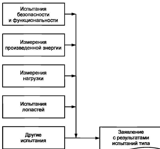
Рисунок 5 — Блок-схема процедуры типовых испытаний
