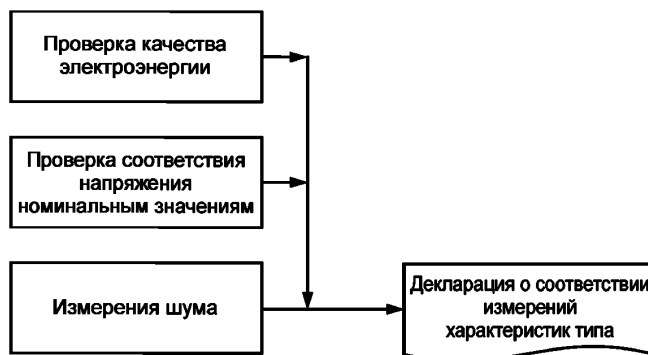
Рисунок 6 — Блок-схема элементов измерения характеристик типа
