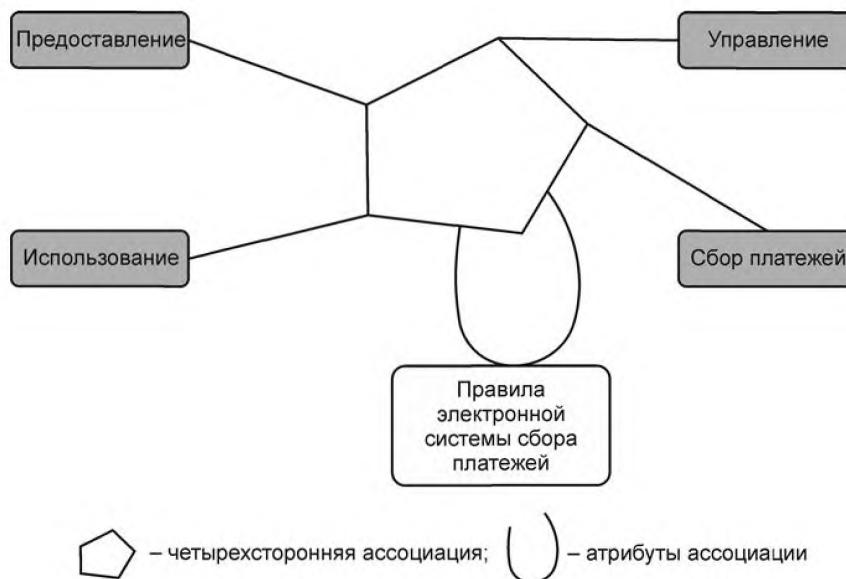
Рисунок 22 — Обнаружение исключений
