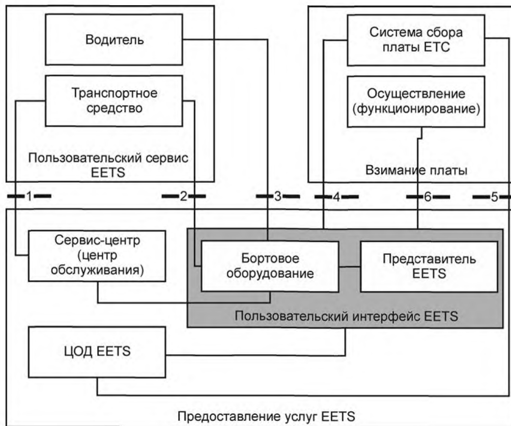
Рисунок D.2 — Архитектура RCI
