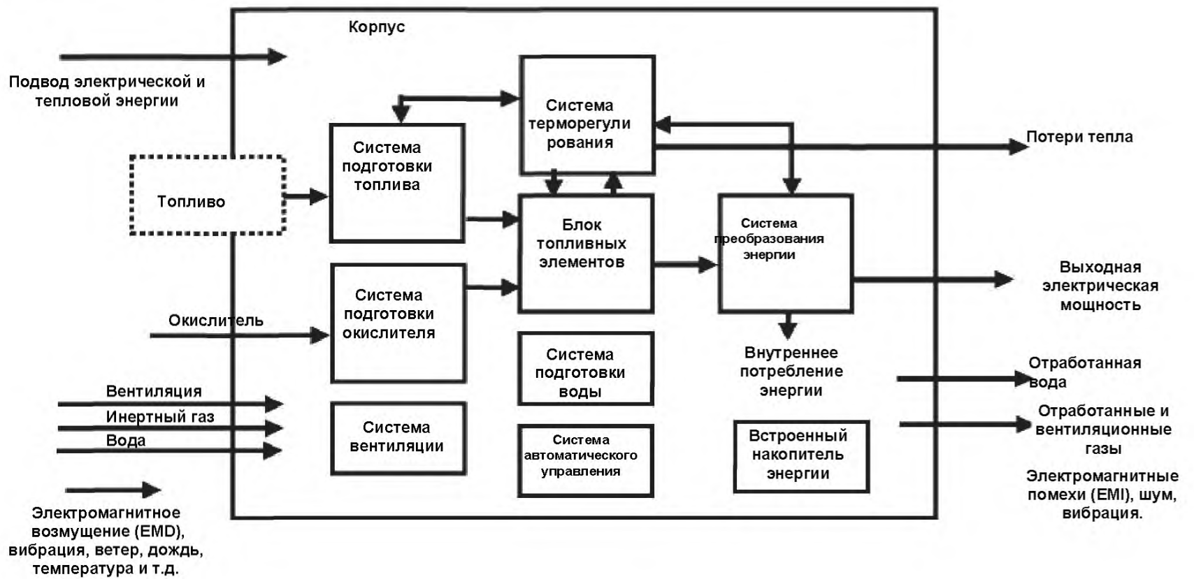
Рисунок 2 – Портативная энергоустановка на топливных элементах (3.49.2)
