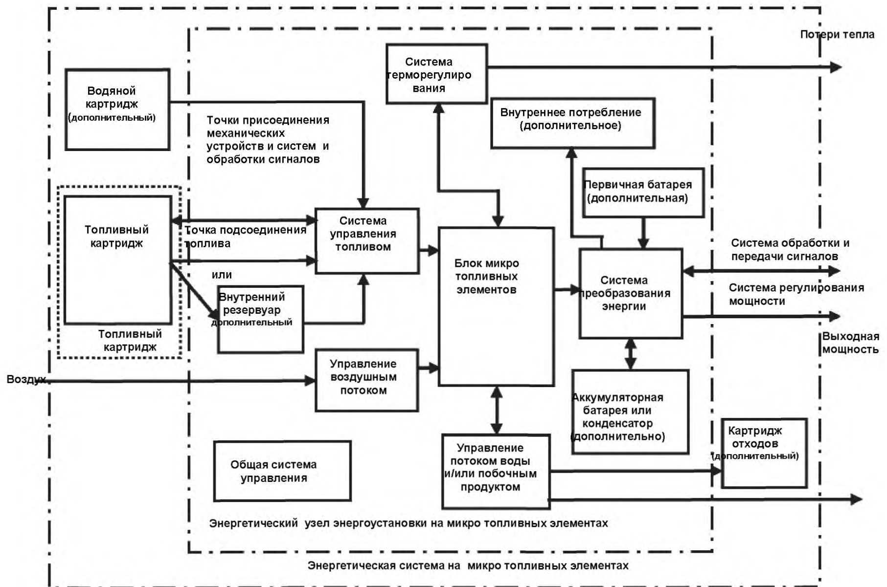
Рисунок 3 – Энергетическая система на микро топливных элементах (3.49.1)
