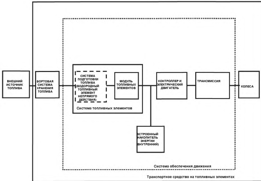
Рисунок 4 – Транспортные средства на топливных элементах (3.51)
