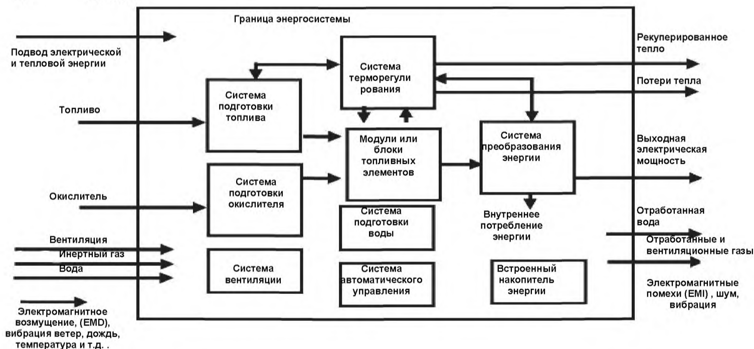
Рисунок 1 – Стационарная энергоустановка на топливных элементах (3.49.3)
