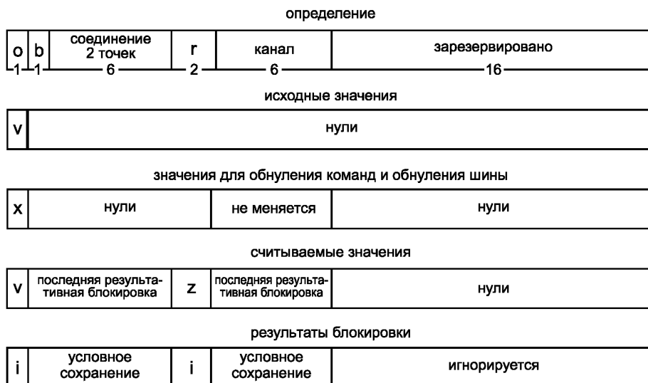
Рисунок 13 — Формат iPCR
