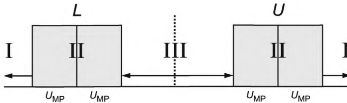
Рисунок 5 — Зона неопределенности (II)
