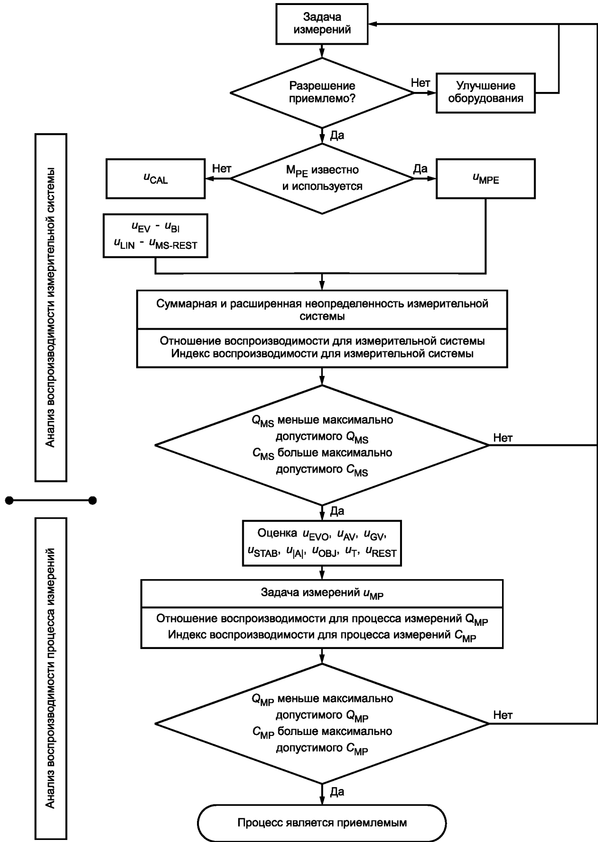
Рисунок 1 — Анализ воспроизводимости процесса измерений и системы измерений
