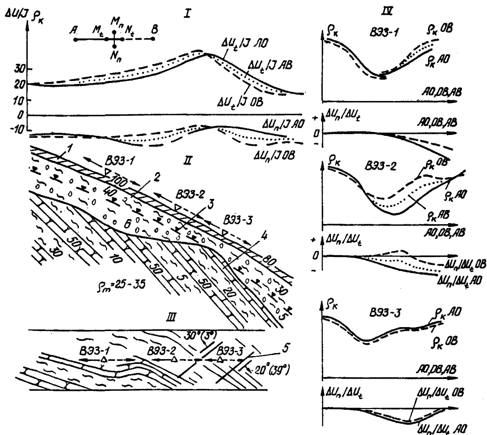
Рис. 3. Геоэлектрическая модель консеквентного оползня I – графики \Delta U_t/I ( \rho_k ), \Delta U_n/I двустороннего трехэлектродного и симметричного ЭП МДС; II – геоэлектрический разрез; III – простираение геоэлектрических границ в плане; IV – кривые \rho_k и \Delta U_n/\Delta U_t двусторонних трехэлектродных и симметричных ВЭЗ МДС; 1 – суглинки и значение их УЭС; 2 – оползневые отложения и значение их УЭС; 3 – положение УГВ; 4 – коренные породы и значение их УЭС; 5 – положение негоризонтальных границ, направление и углы падения
