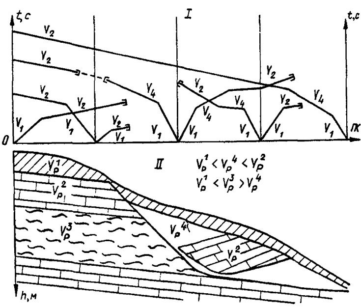
Рис. 5. Геосейсмическая модель консеквентного и инсеквентного оползней I – система встречных и нагоняющих годографов над ними; II – геосейсмический разрез
