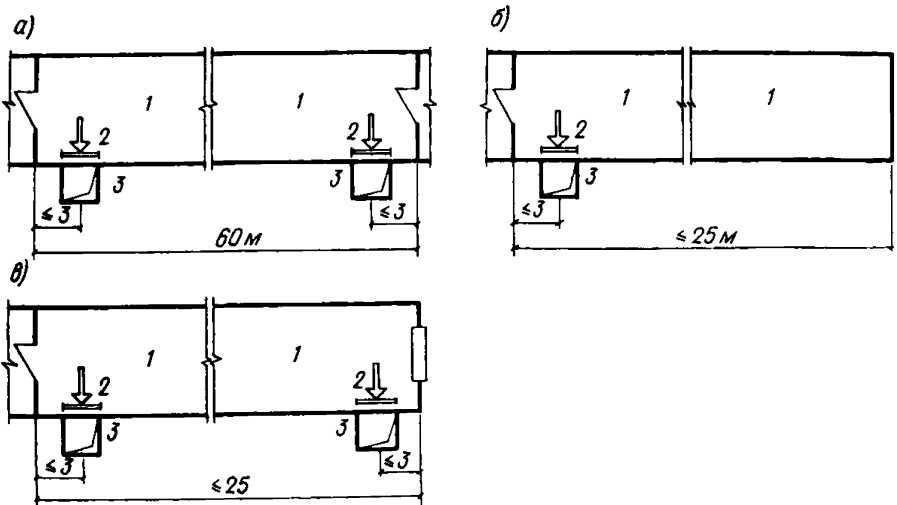
Рис. 2. Размещение клапанов дымоудаления в поэтажном коридоре (план) а – промежуточный отсек коридора; б и в – тупиковые коридоры без естественного освещения и с естественным освещением; 1 – коридор; 2 – клапан дымоудаления; 3 – шахты дымоудаления
