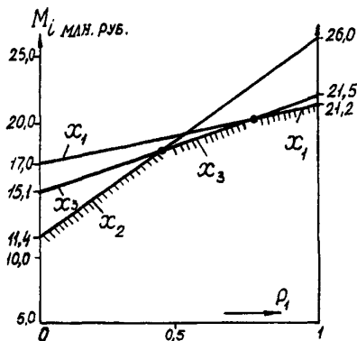
Рис. 2. Зависимости математических ожиданий затрат для разных вариантов решения от вероятности реализации условий Y_1 .
