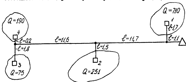
Рис. 1. Расчетная схема системы теплоснабжения.
