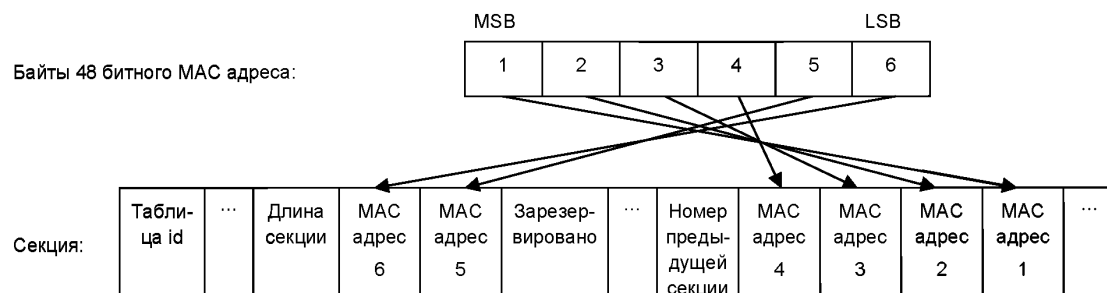
Р и с у н о к 4 — Отображение байтов MAC адреса в полях секции
