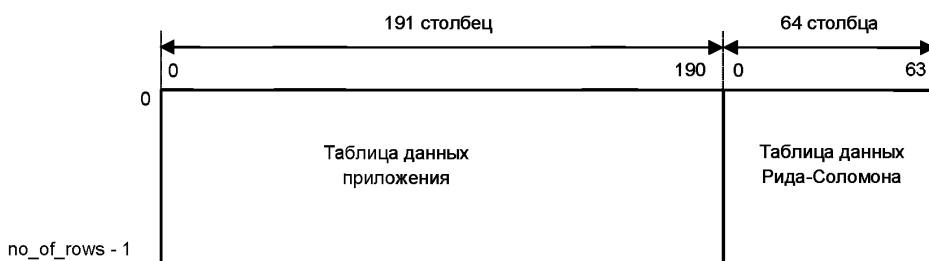
Р и с у н о к 8 — Структура кадра MPE-FEC
