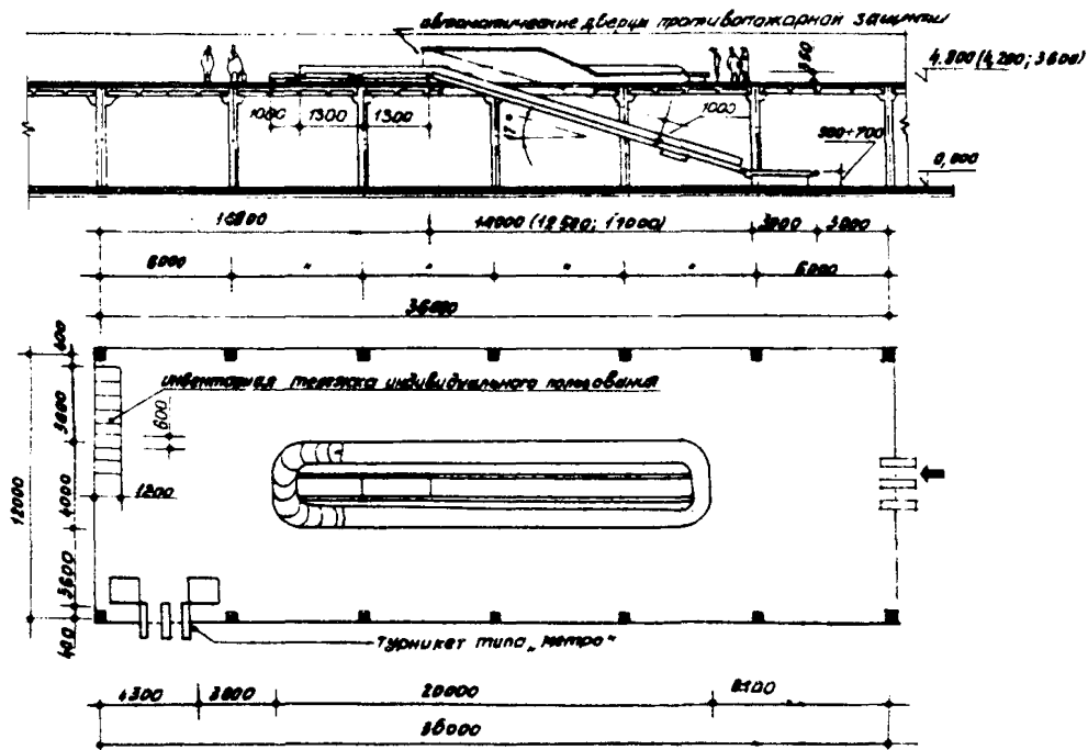
Рис. II. Схема планировки зоны выдачи багажа пассажирам, прилетевшим самолетом Ил-62 (два технологических уровня с подачей багажа с нижнего уровня)
