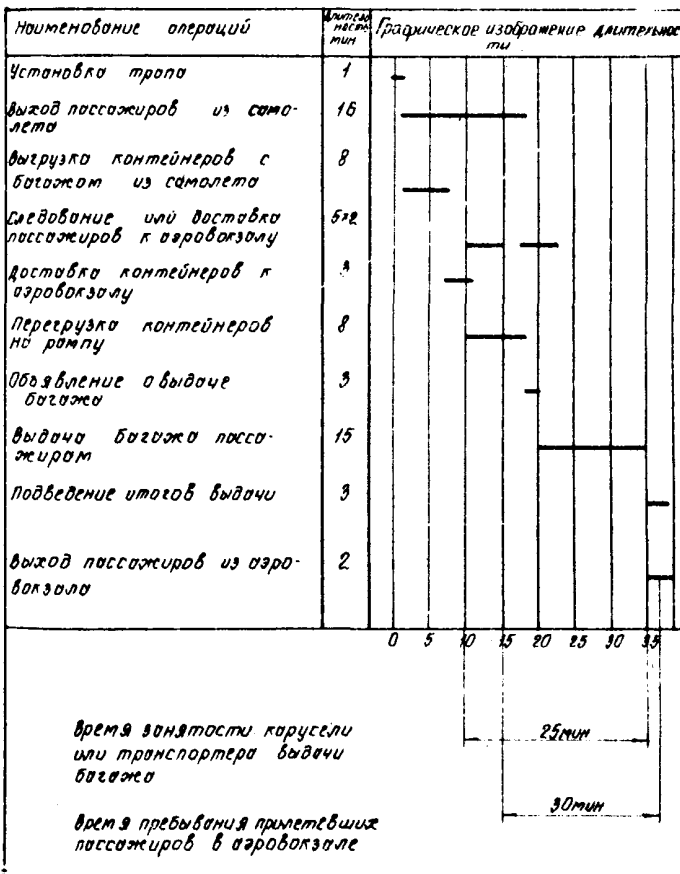
Рис. 14. Технологический график обслуживания прилетевших пассажиров, обработки багажа самолетов Ил-86
