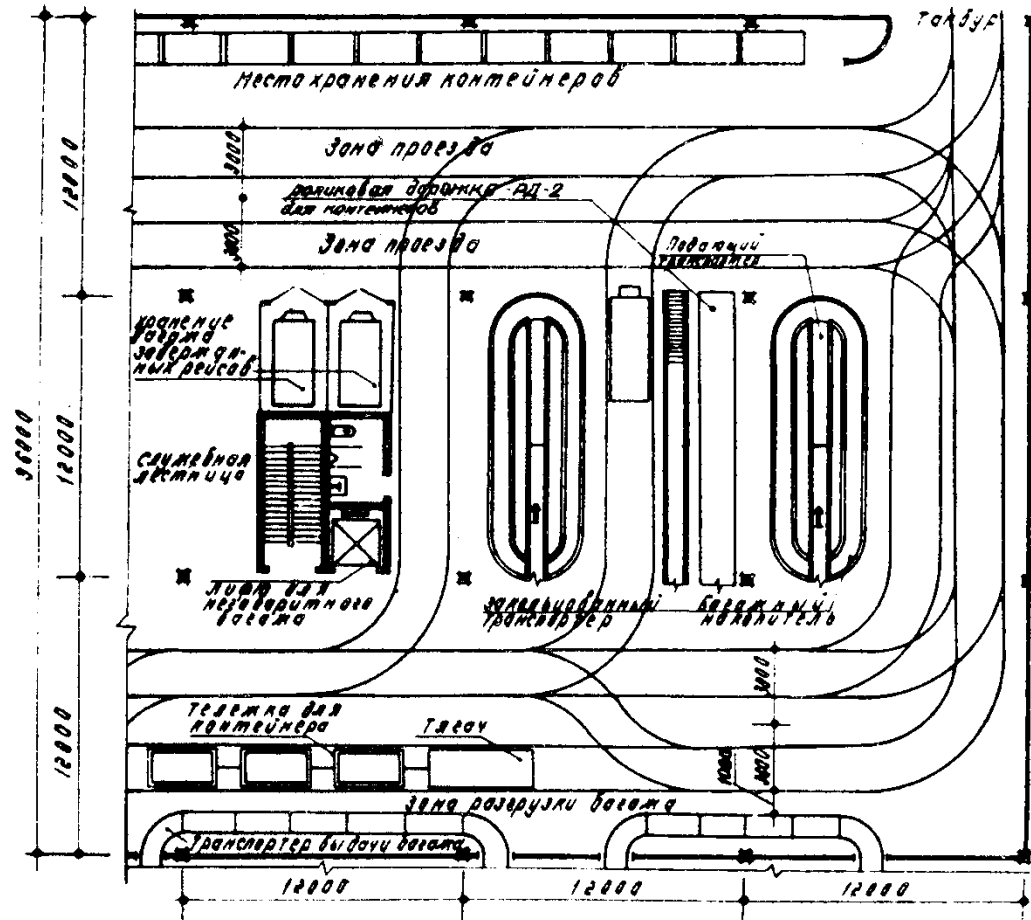
Рис. 10. Схема планировки зоны обработки багажа (два технологических уровня)
