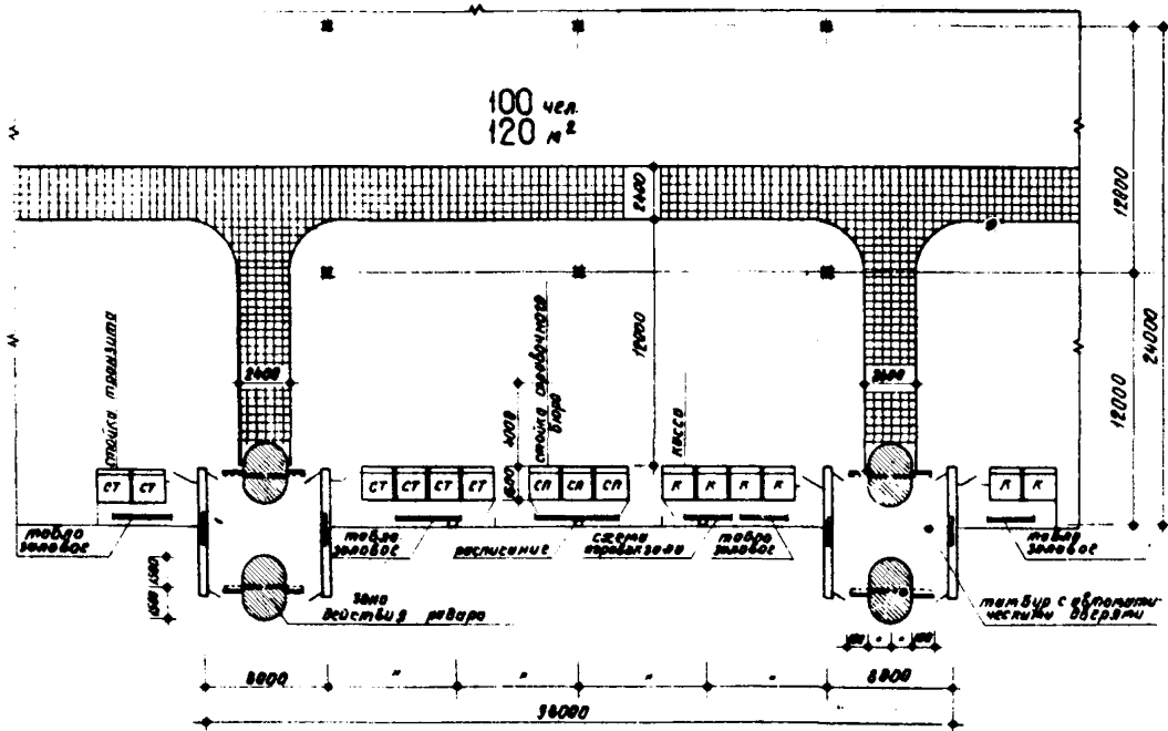
Рис. 5. Схема планировки вестибюля (аванзал и справочно-информационная зона) больших аэровокзалов
