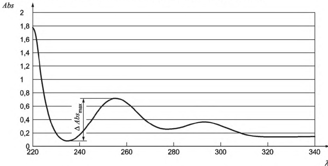
Рисунок 1 — Пример спектра раствора В на фоне раствора А для определения содержания фенольного гидроксила лигносульфонатов, показывающий максимум и минимум (в случае подсчета с левой стороны) поглощения
