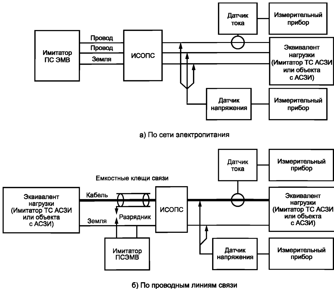
Рисунок Б.1 — Типовые схемы измерений параметров испытываемых средств обнаружения преднамеренных силовых электромагнитных воздействий с имитаторами преднамеренных силовых электромагнитных воздействий
