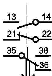
Три контактных элемента
