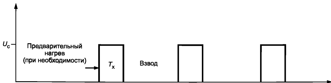
Профиль напряжения управления U_c
