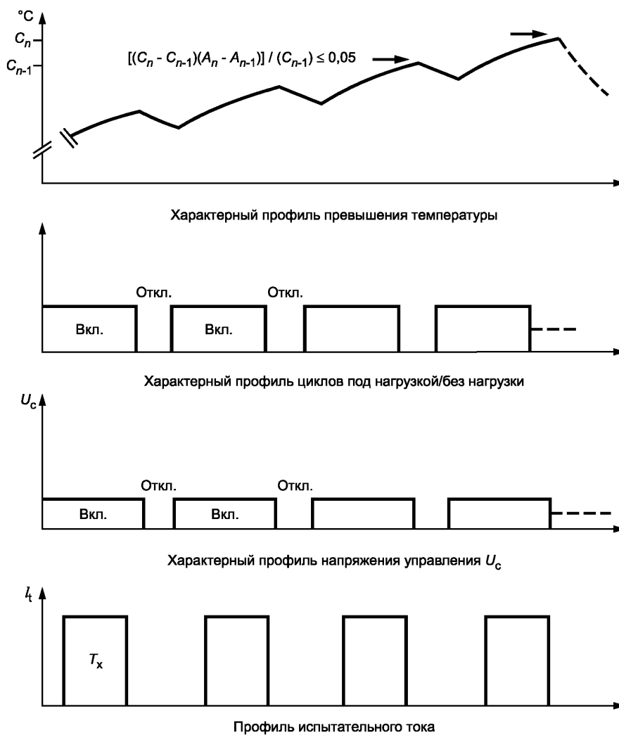
Рисунок F.1 — Профиль испытания на тепловую стабильность
