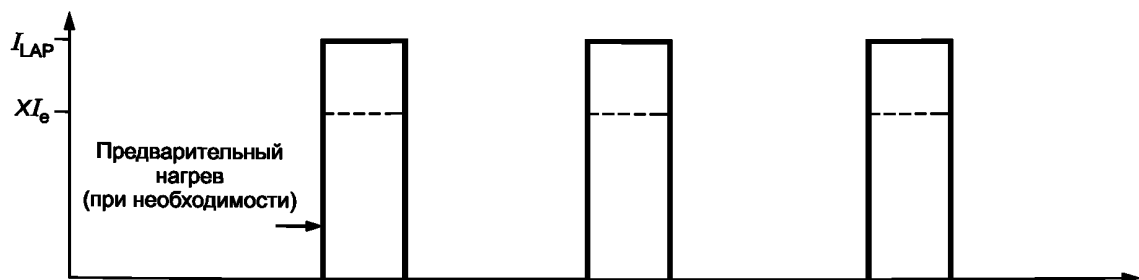
Профиль испытательного тока
