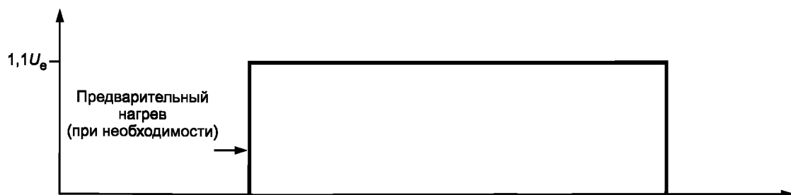
Профиль испытательного напряжения U_T главной цепи
