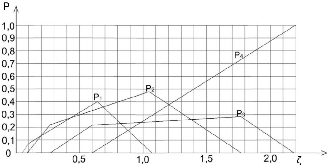
Рисунок 4.1 - Вероятности различной степени разрушения здания (сооружения) и повреждения технологического оборудования в зависимости от величины обобщенного показателя устойчивости, \xi_{30}(\xi_{70})
