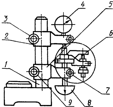
1—стойка; 2—дополнительный кронштейн; 3, 7, 9—зажимной винт; 4—поверяемый микатор; 5—кронштейн; 6—установочное приспособление; 8—оптикатор 01П или 02П, или 06П по ГОСТ 10593—74
