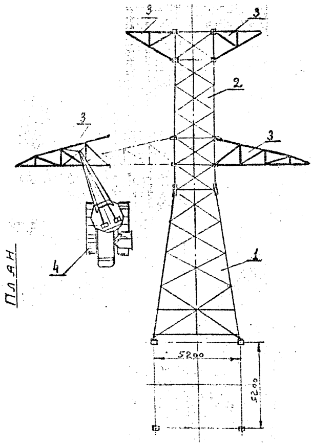
Рис 63 Пристыковка траверсы к стволу опры 4220-3
