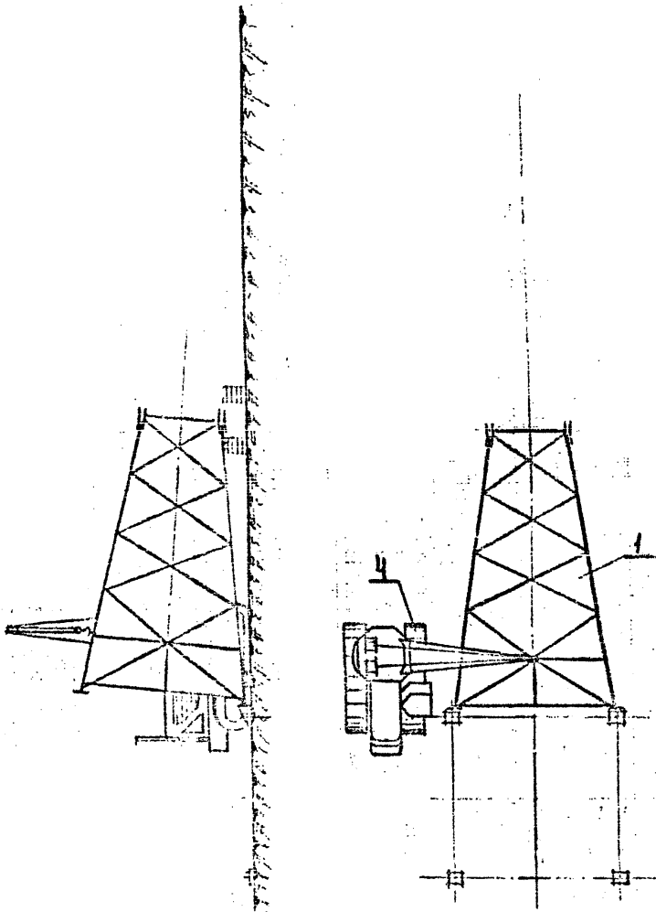
Рис. 6 Сборка 1 ой секции ствола опоры 4220-3
