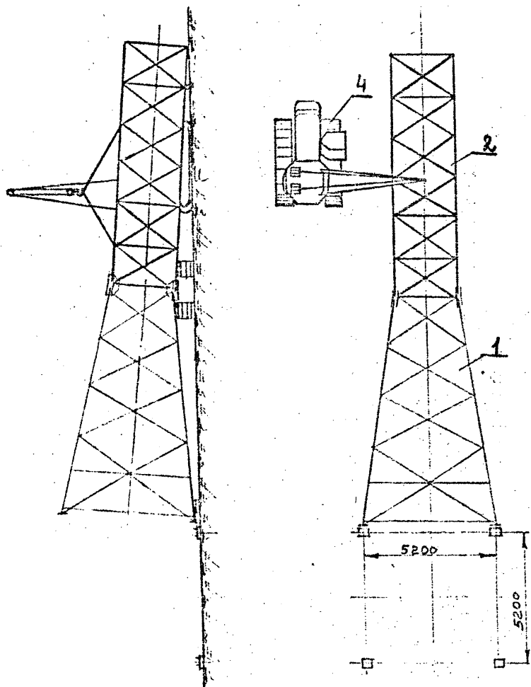
Рис. 62 Пристыковка 2 ой секции ствала опоры 4220-3
