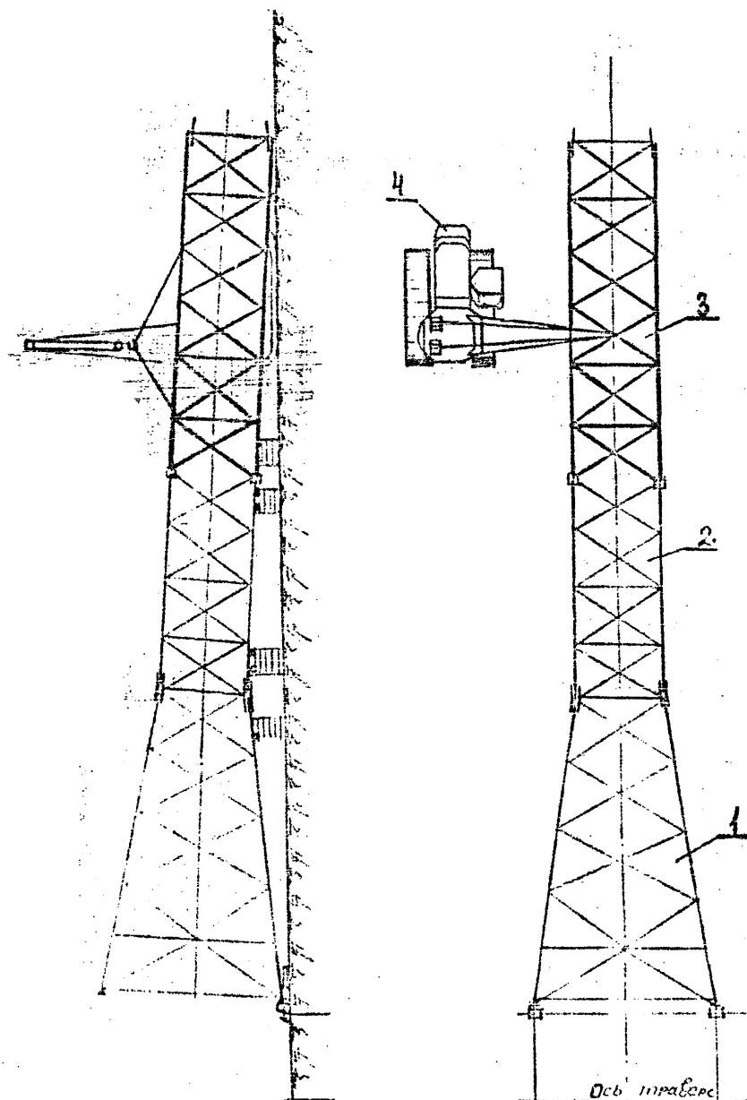
Рис. 51 Пристыковка 3ей секции ствола опоры 4220-2
