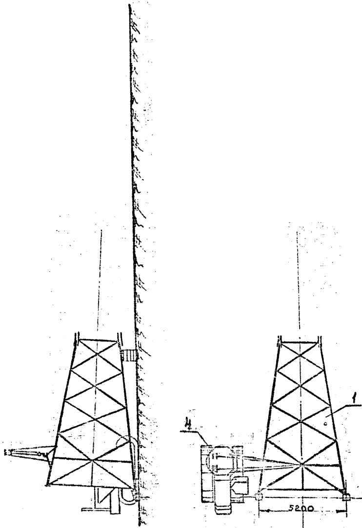
Рис. 49 Сборка 1 ой секции стб. оп. У220-2.
