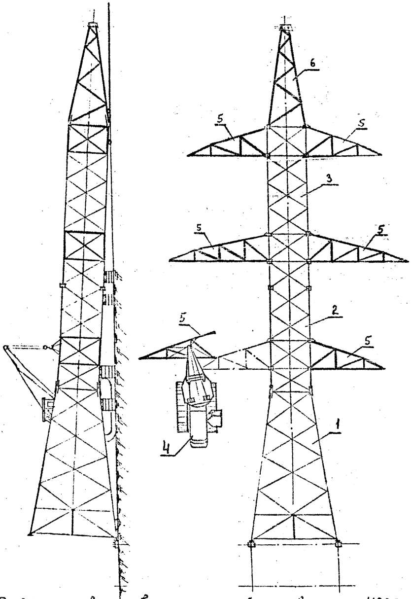
Рис. 8. Пристыковка траверс и тросостойки к стволу опоры У220-2
