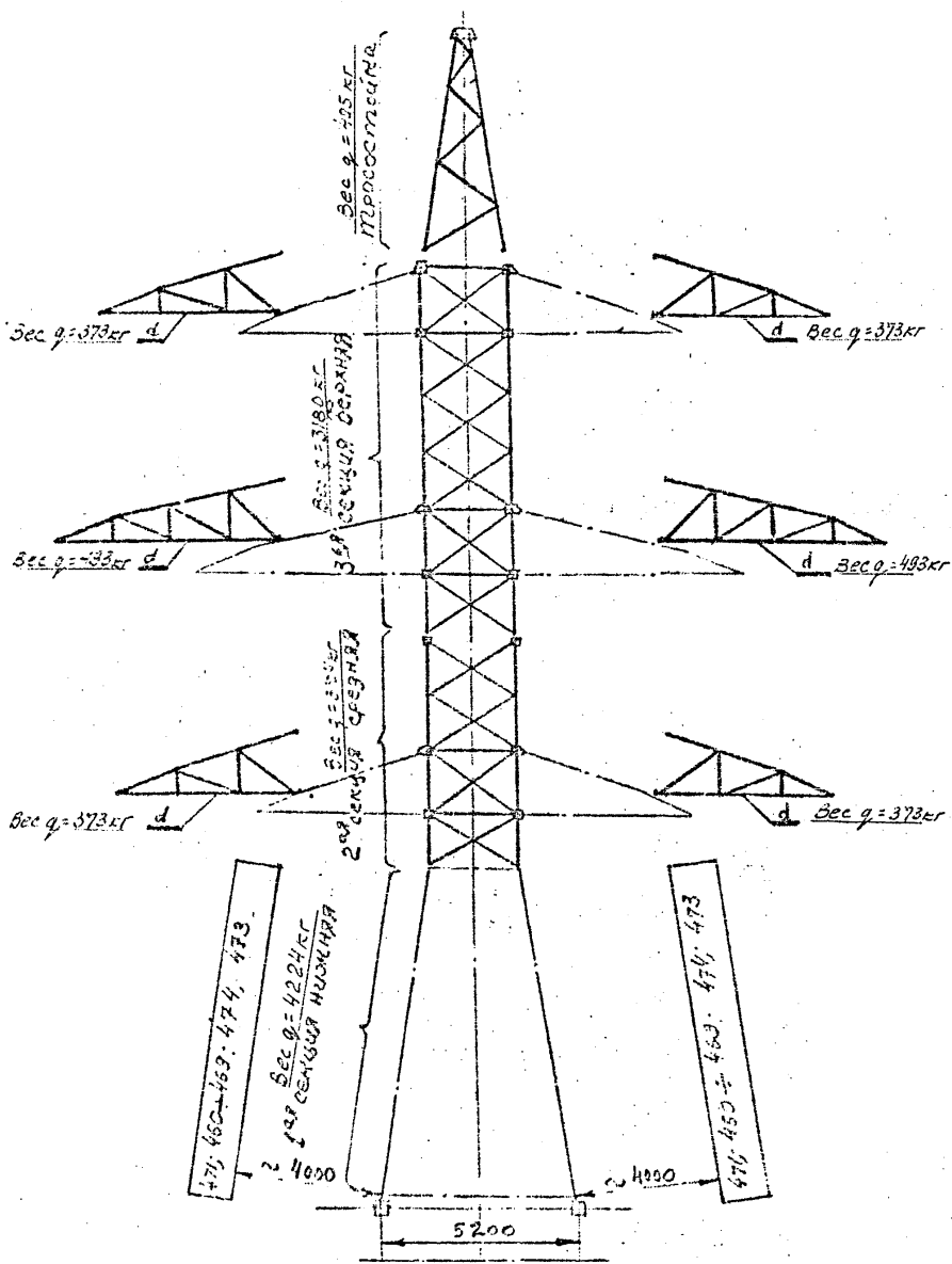
Рис. 46. Разкладка пакетов и секций опоры У220-2 на пикете:
