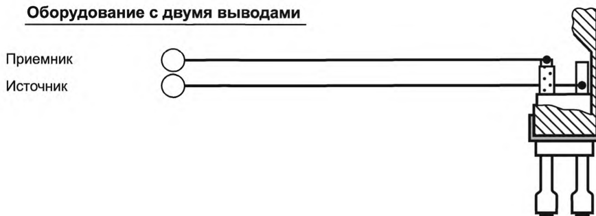
Рисунок 2 — Соединение датчика с измерительным оборудованием
