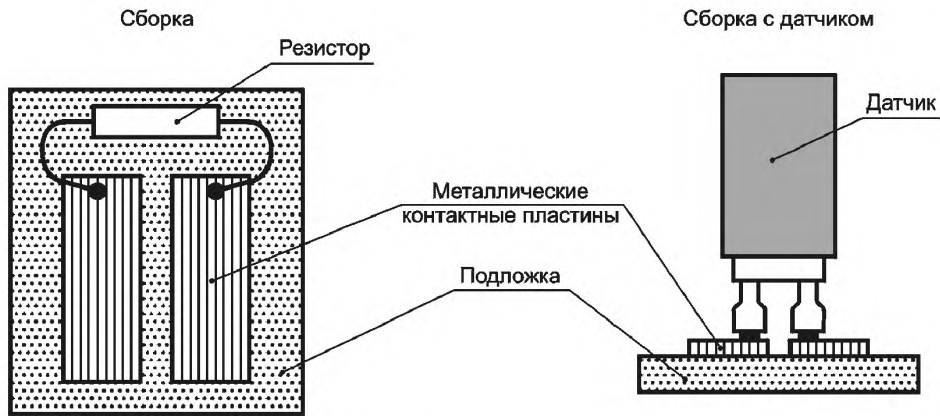
Рисунок 3 — Сборка для проверки сопротивления
