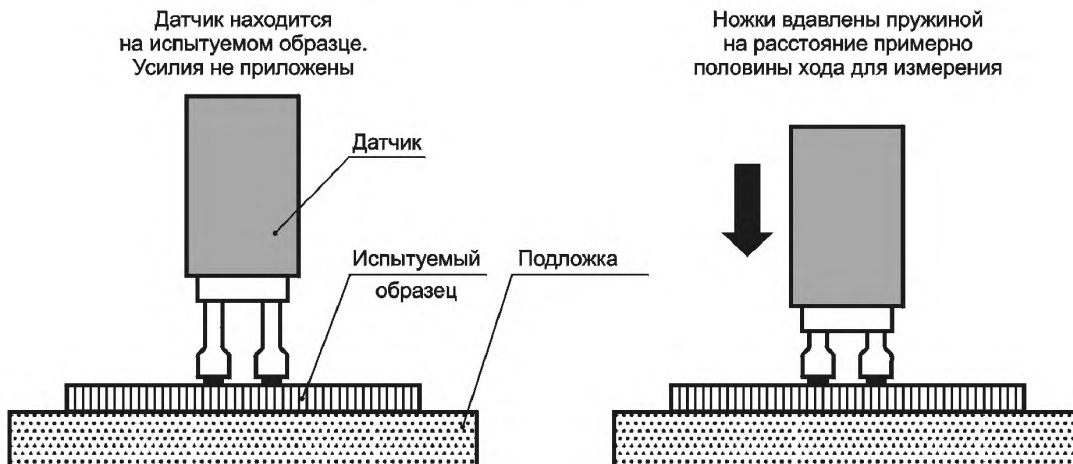
Рисунок 4 — Сжатие пружин при измерении
