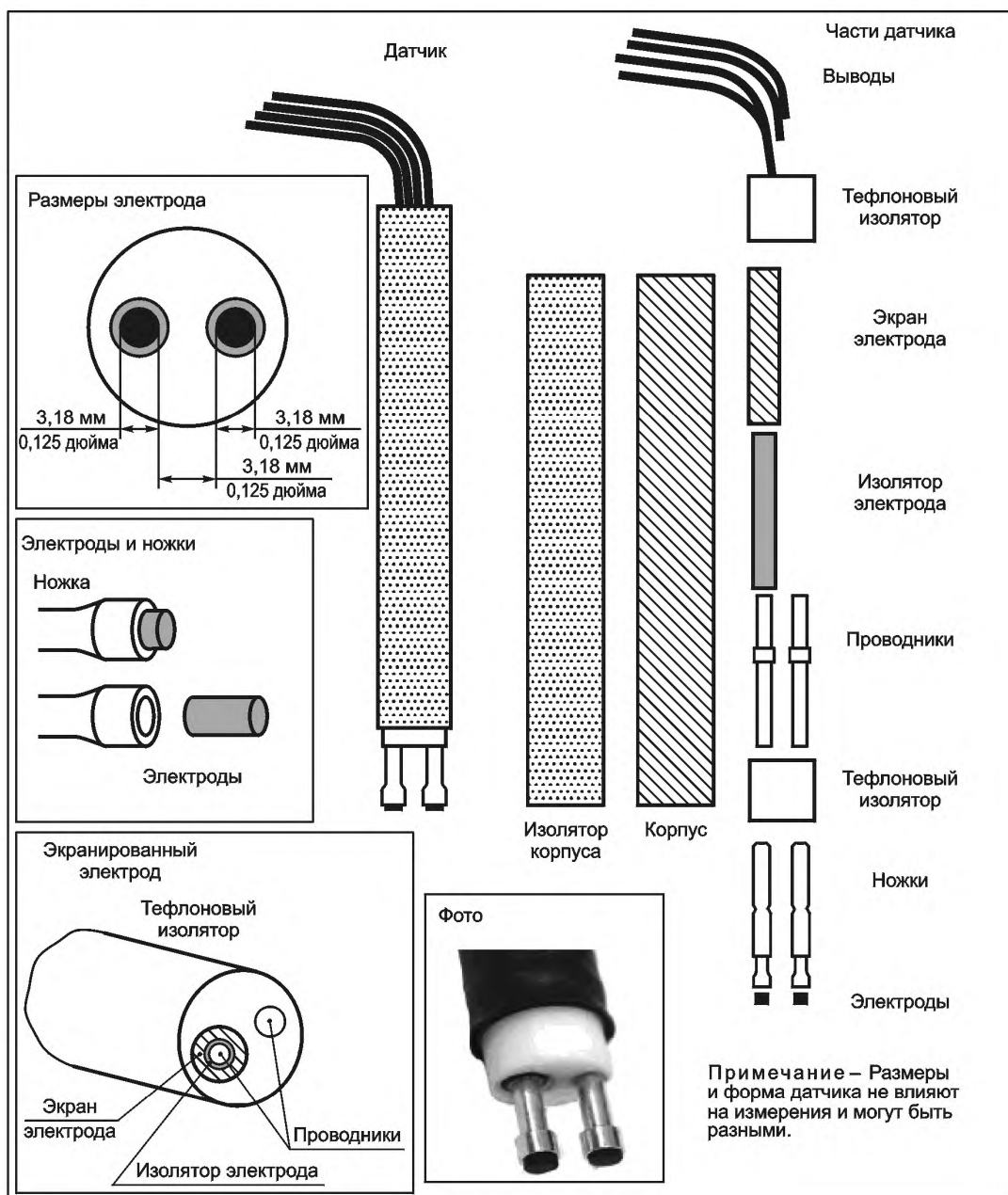
Рисунок 1 — Конфигурация двухконтактного датчика
