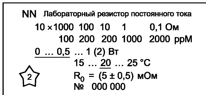
Рисунок 3 — Пример маркировки пятидекадного резистора
