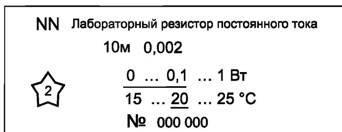
Рисунок 2 — Пример маркировки единичного резистора
