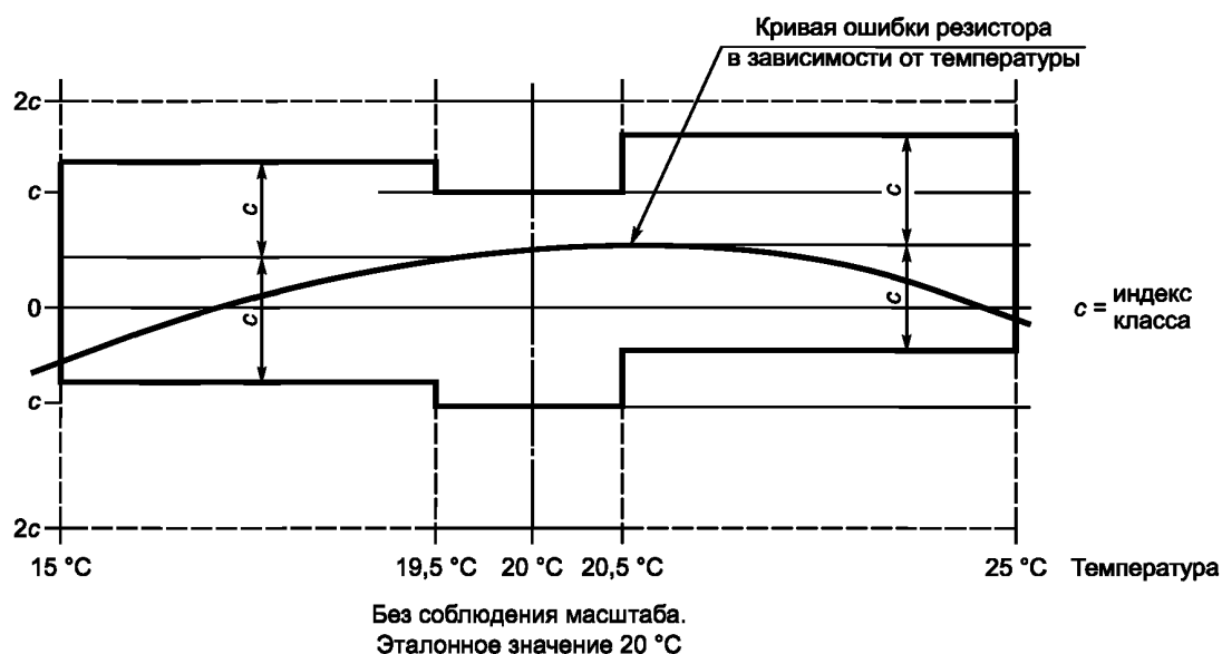
Рисунок 1 — Влияние температуры
