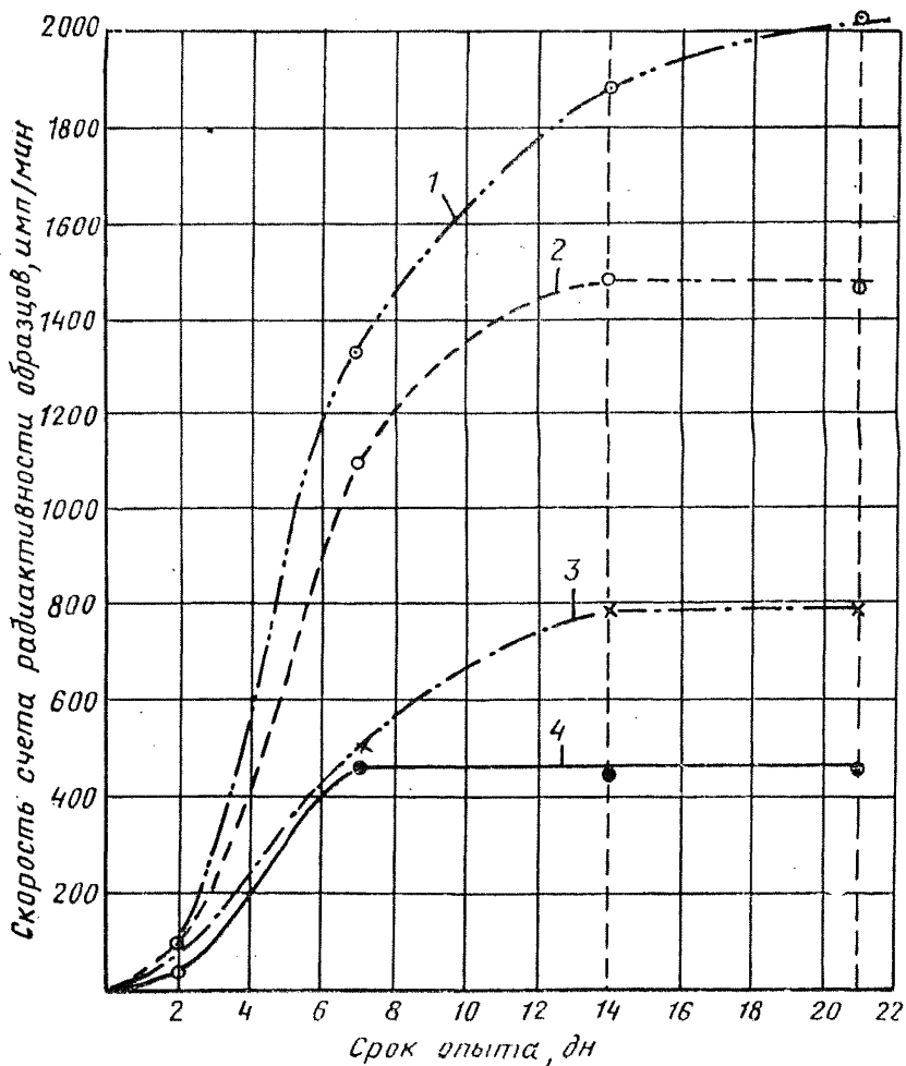
Рис. 69. Зависимость пропускания P^{32} от породы древесины и длительности биологических испытаний (Ф. Ф. Мазур, Мгуен Куанг)
