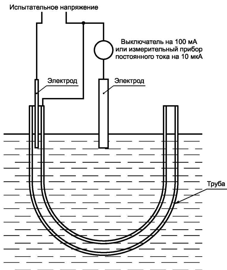
Рисунок 5 — Установка для испытаний электрической прочности и сопротивления изоляции. Гибкие трубы и трубы повышенной гибкости
