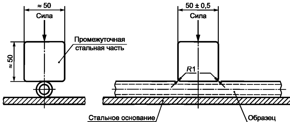
Рисунок 1 — Установка для испытаний на сжатие
